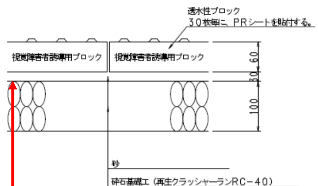
千葉市道路施設標準図 (道路付属施設工) 抜粋
