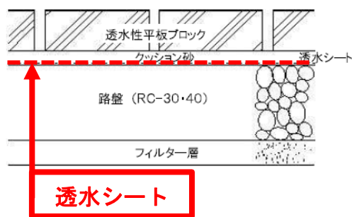
千葉市歩行空間整備マニュアル抜粋
