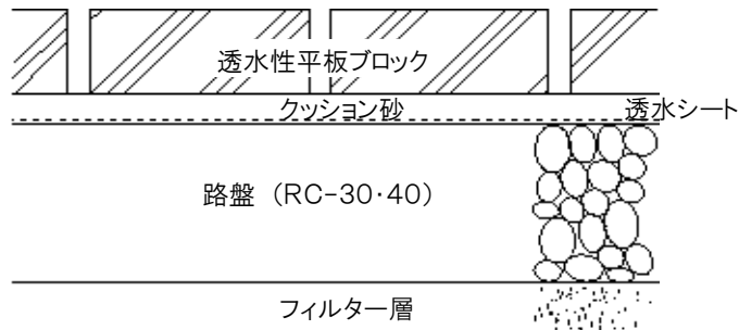
図26 透水性平板ブロック舗装の構造図
