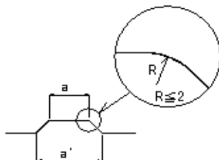
図33 ハーフドーム型の突起詳細
