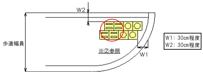
図39 交差点部(歩道が狭い場合)
