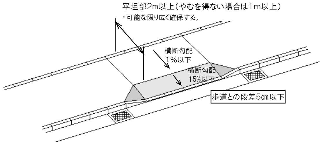
図21 歩道内においてすりつけを行う構造
