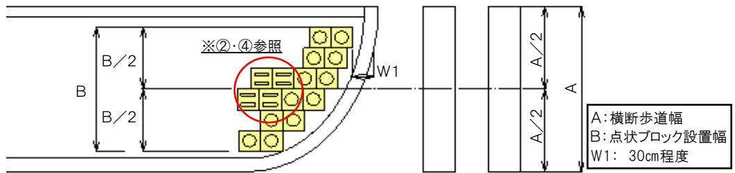
図40 交差点部(歩道が狭い場合)
