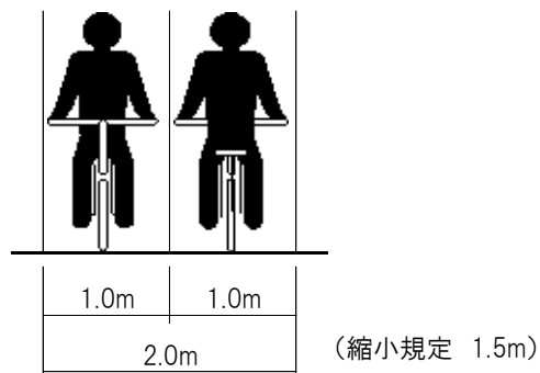
図5 第3種及び第4種の自転車道幅員の考え方
