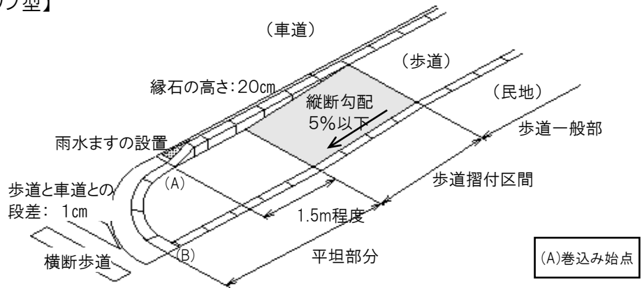
図13-1 横断歩道接続部等における構造(植樹帯等がない場合)
