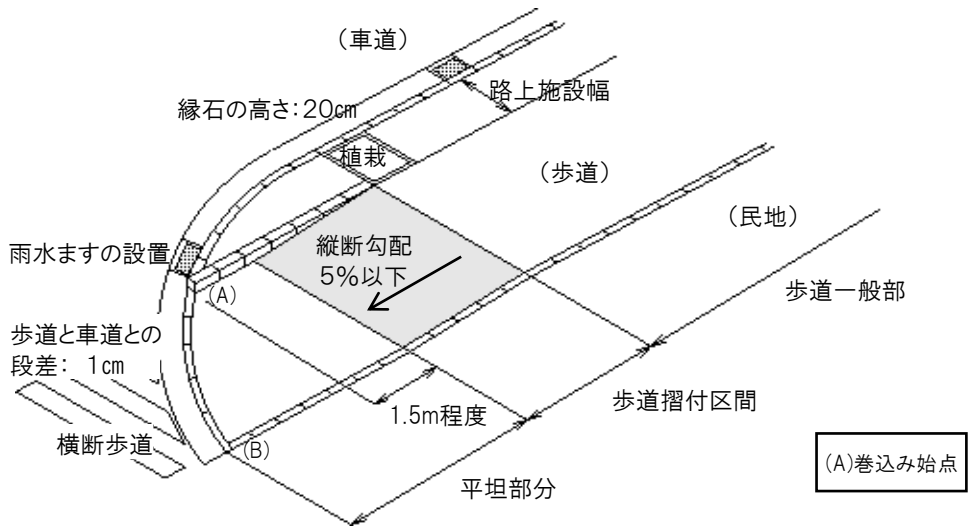
図13-2 横断歩道接続部等における構造(植樹帯等がある場合)
