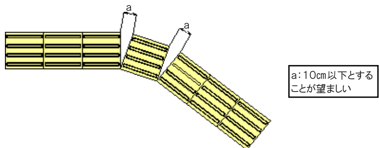
図45 屈曲部の設置例
