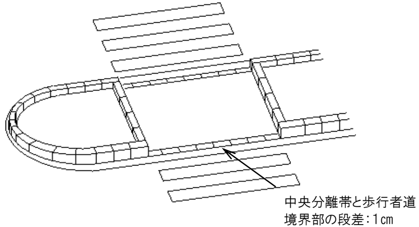
図17 歩道箇所における構造(中央分離帯等がある場合)
