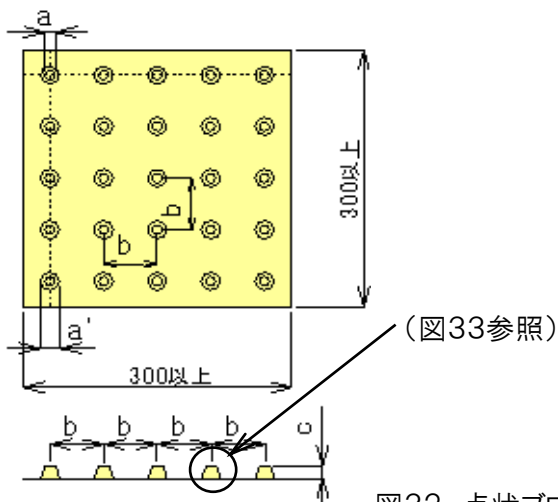
図32 点状ブロックの形状・寸法及び配列
