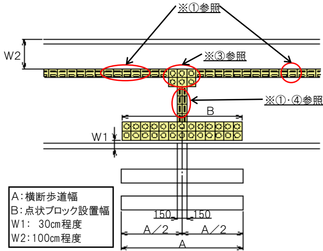
図37 単路部(歩道が広い場合)
