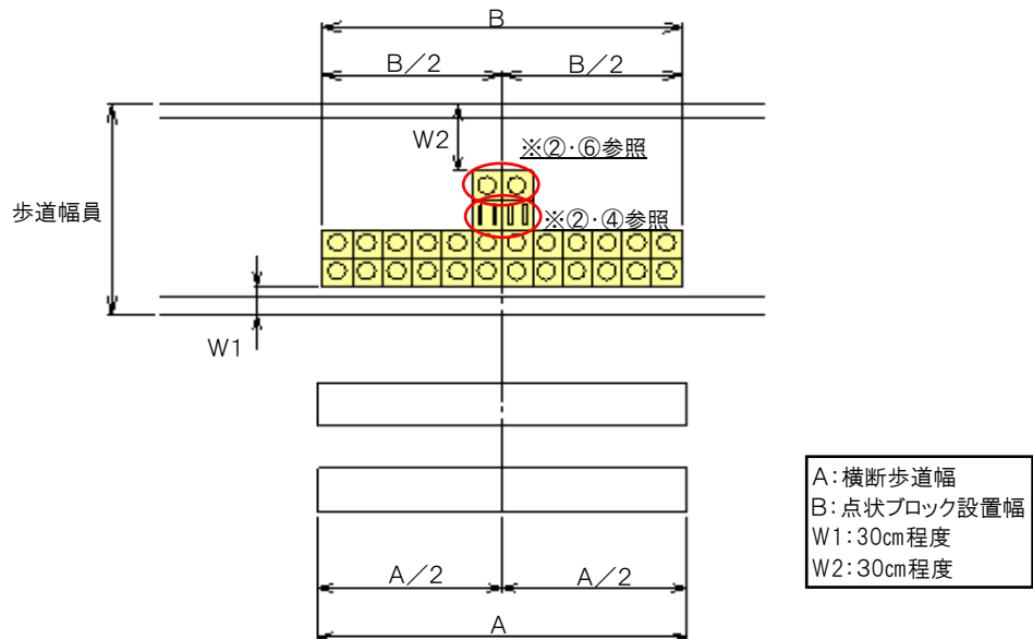
図42 単路部(歩道が狭い場合)
