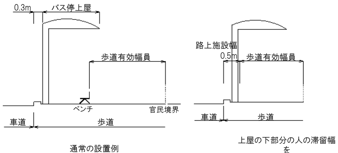
図7 上屋を設ける場合の歩道幅員
