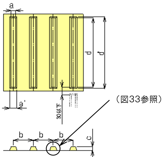
図31 線状ブロックの形状・寸法及び配列
