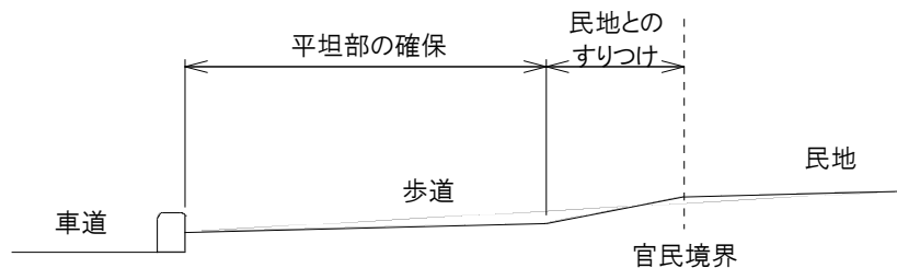
図18 歩道と民地のすりつけ
