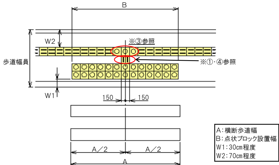
図41 単路部(歩道が狭い場合)
