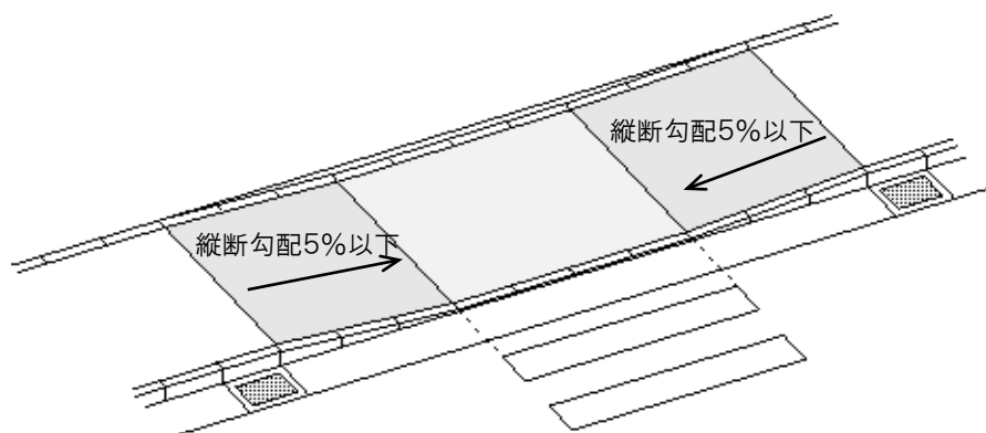
図16 歩道箇所における構造(交差点部以外に横断歩道がある場合)
