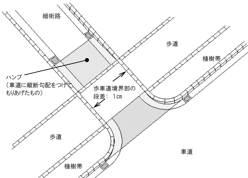
図23 切り開き形式でハンプを設置した場合
