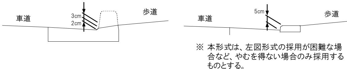
図19 セミフラット形式及びマウンドアップ形式の縁石の構造
