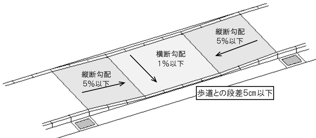
図22 歩道の全面切り下げを行う場合
