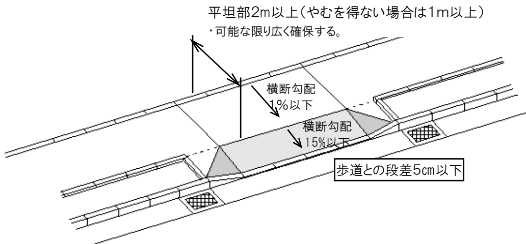
図20 植栽帯等の幅員内ですりつけを行う構造
