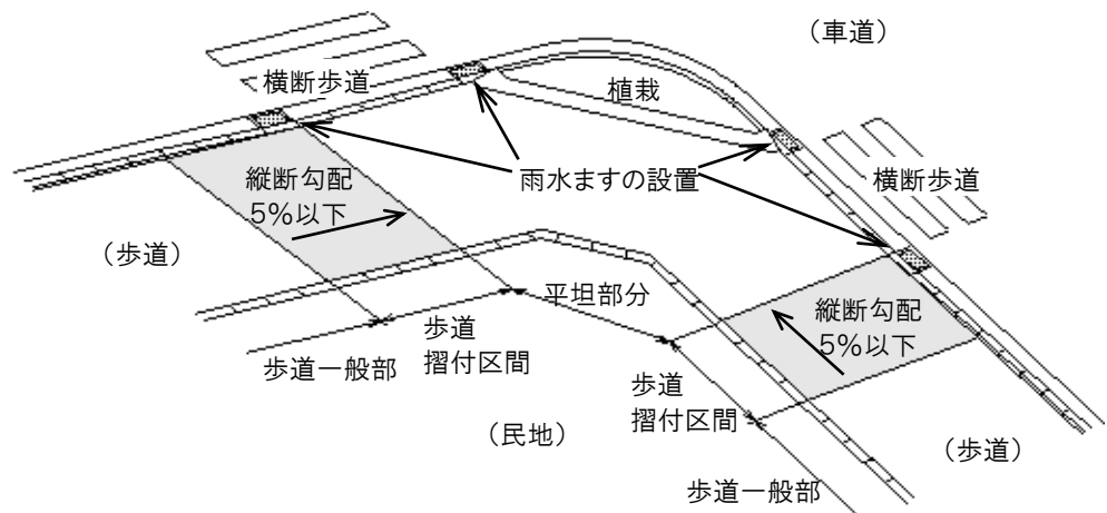
図12-3 横断歩道接続部等における構造(交差点に横断歩道がある場合)
