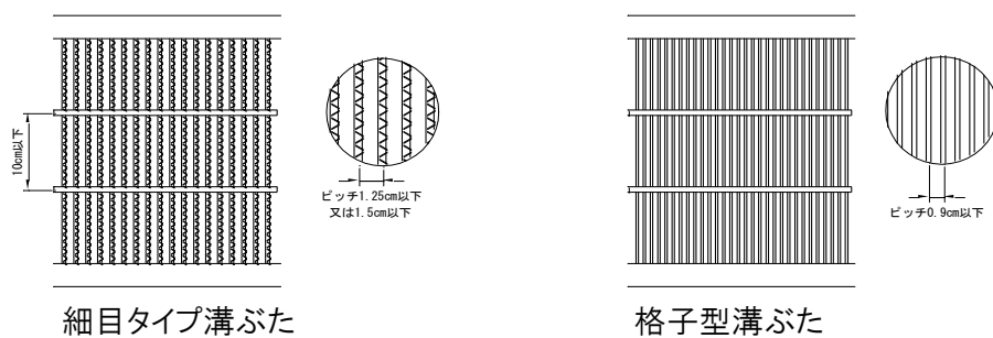
図29 溝ぶたの例
