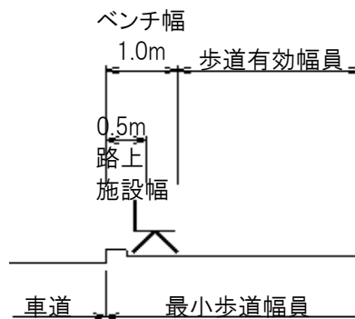
図6 ベンチを設ける場合の歩道幅員
