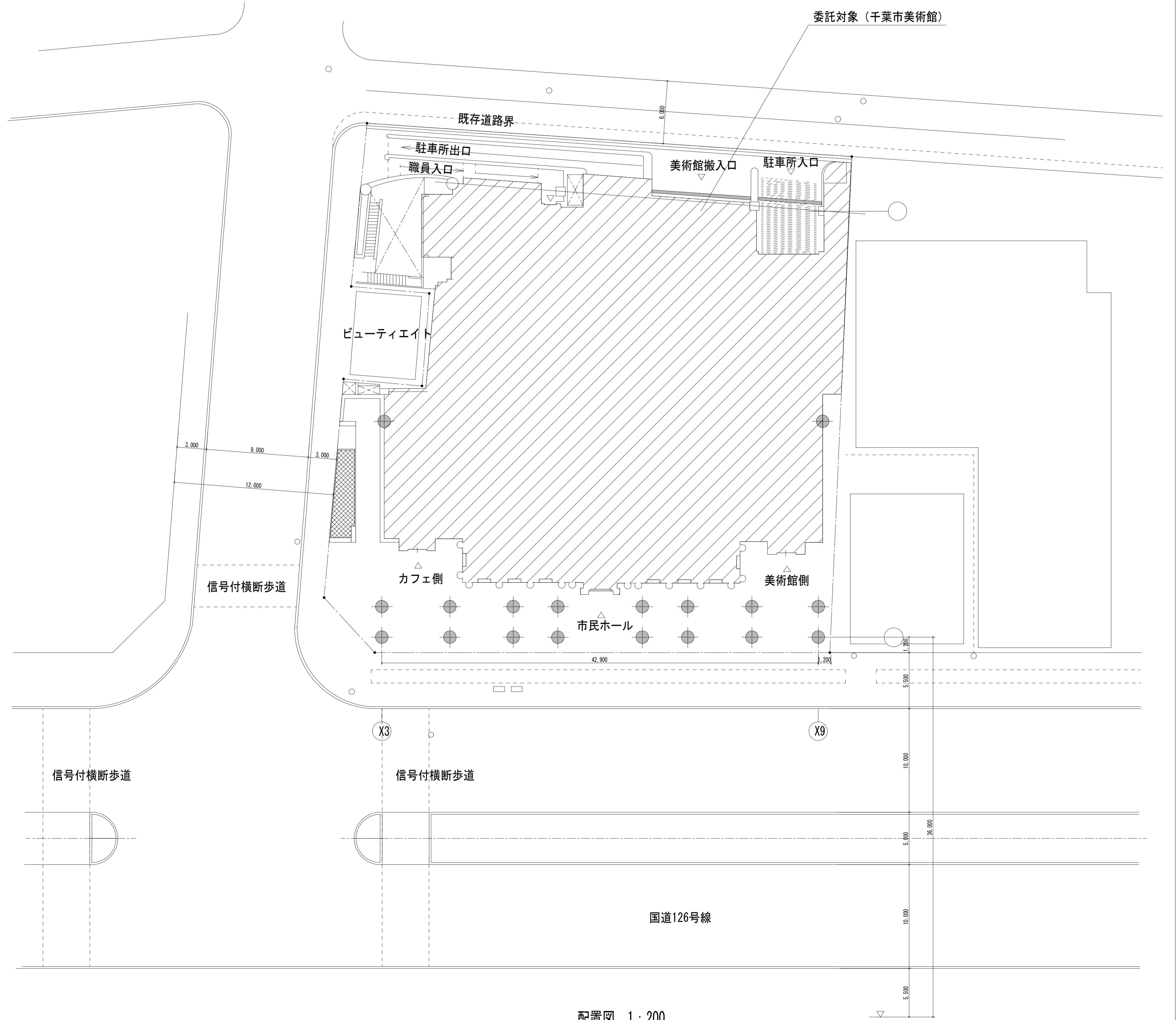
配置図 1 : 200
