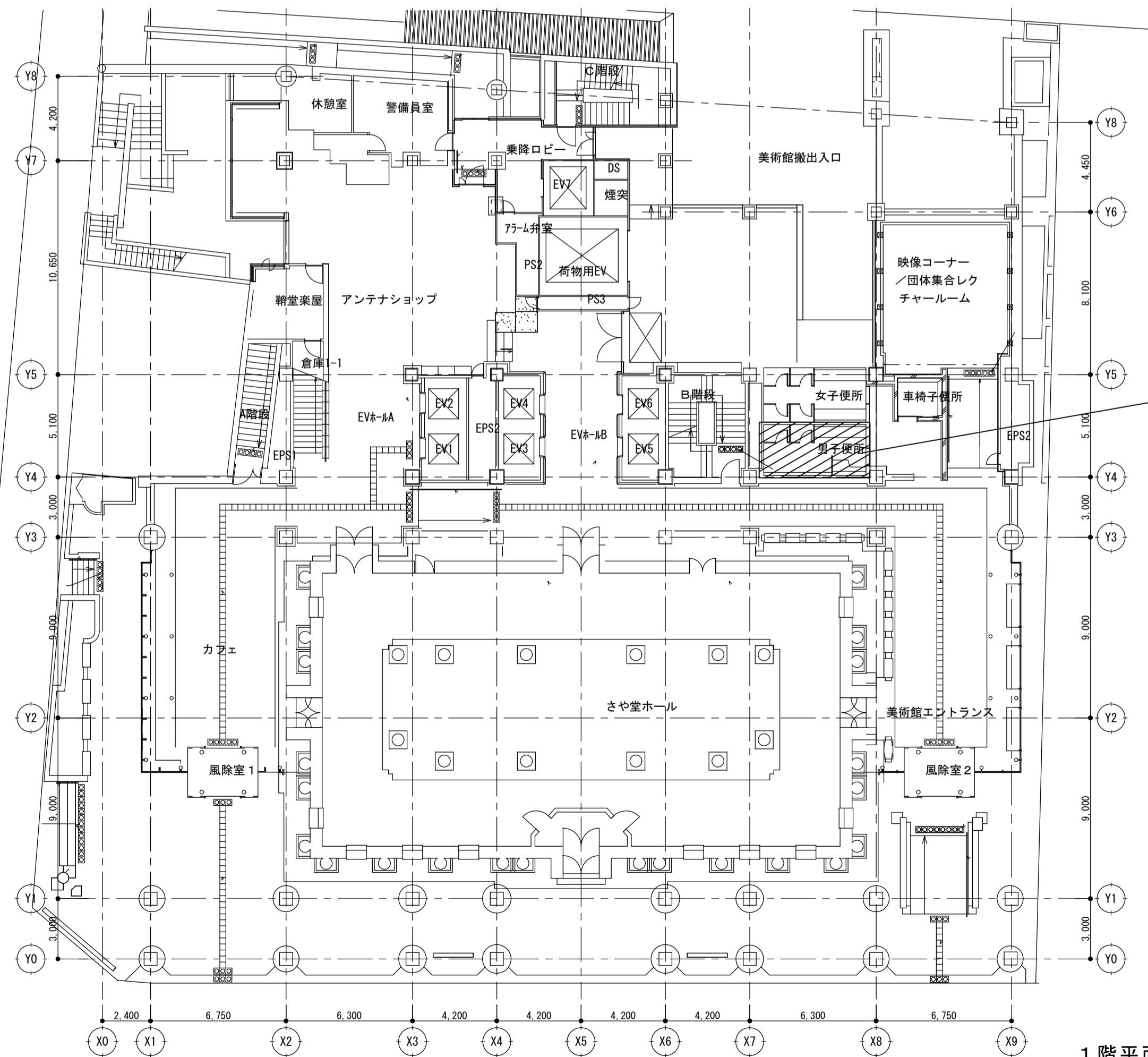
1階平面図
