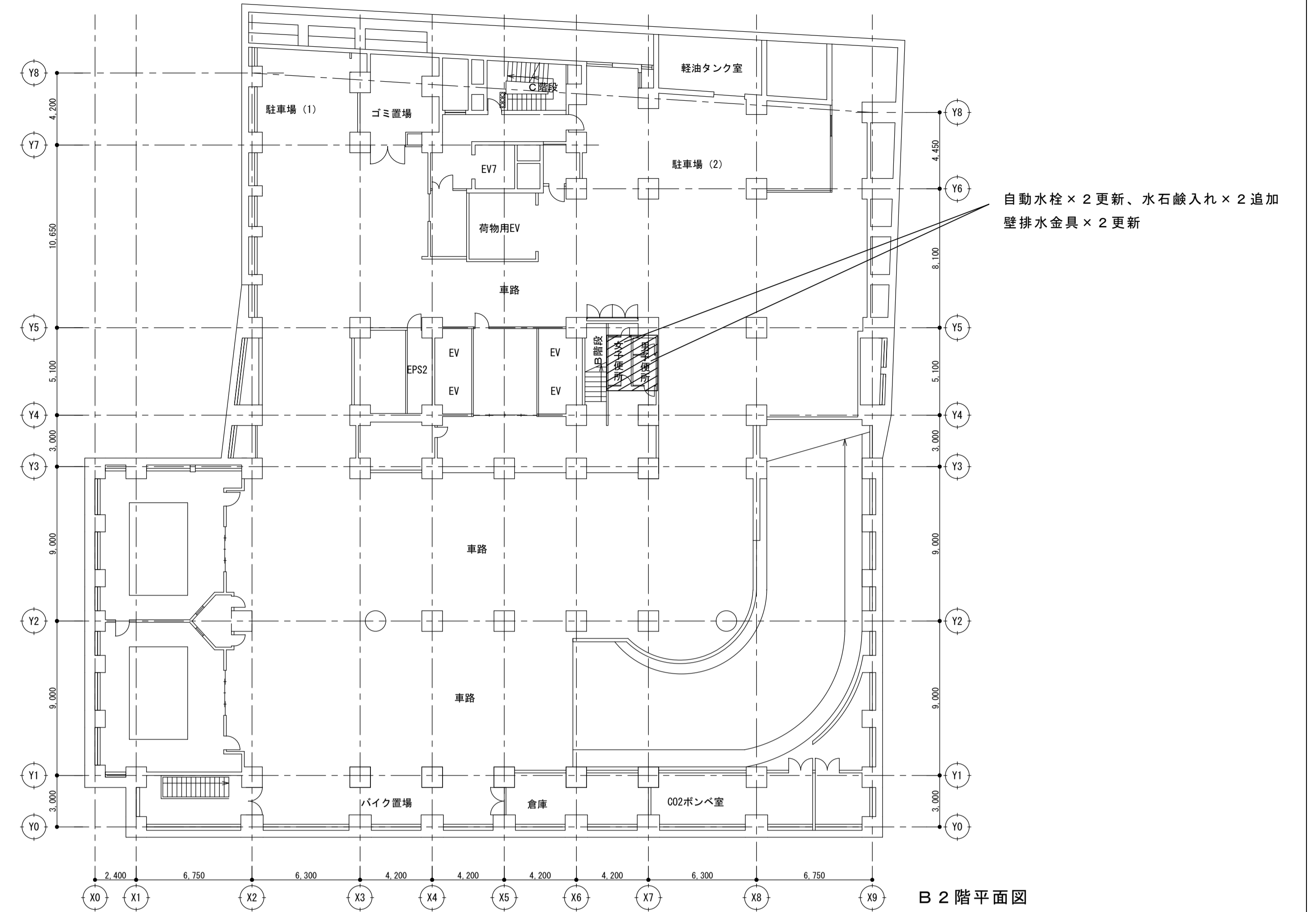
B2階平面図
