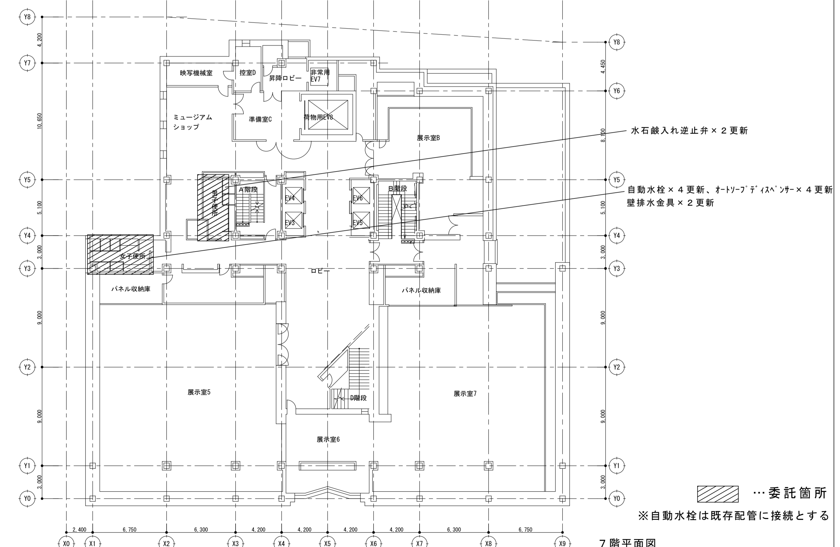
7階平面図
