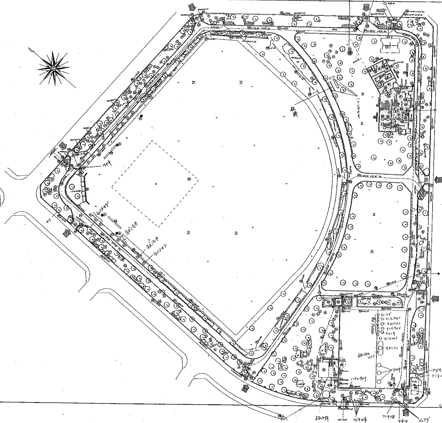
公園名 一本松公園 図面名 平面図 縮尺 1:300 作成年月日 昭和59年3月 千葉市公園管理課
