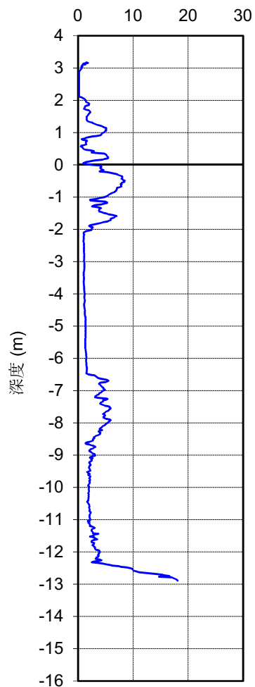
換算N値
