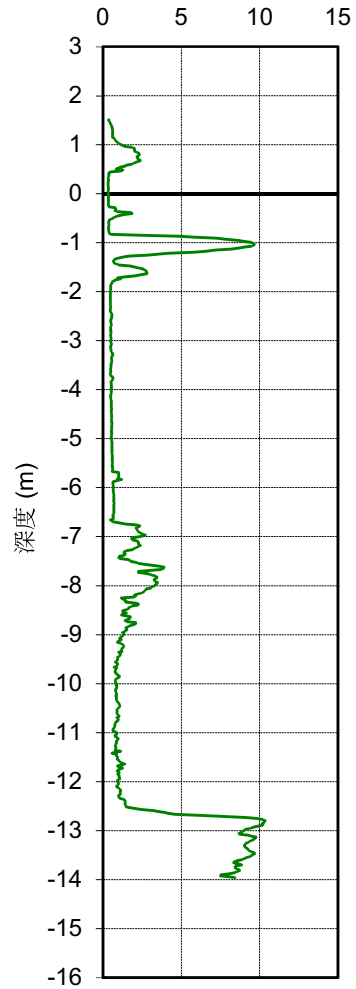
補正先端抵抗 qt (Mpa)
