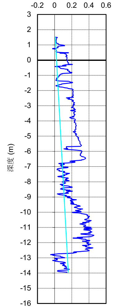
間隙水圧 u (Mpa)
