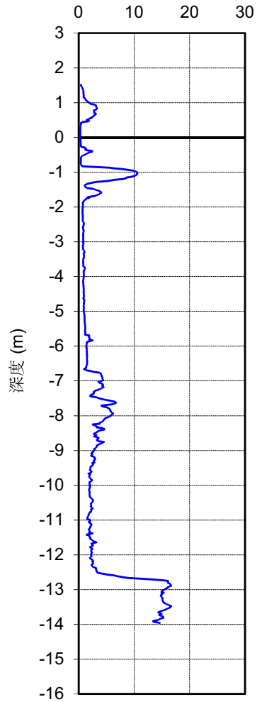
換算N値
