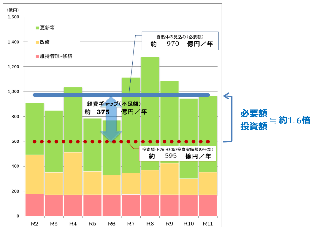
■図表 2-15 耐用年数経過時に単純更新した（自然体の）見込み（10年間）
