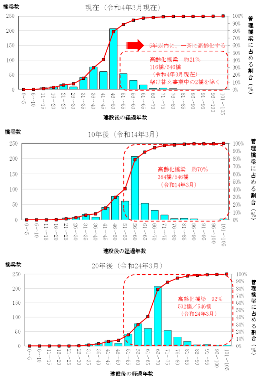
■図表 2-12 橋梁の例 架設後経過年数別の橋梁数の分布
