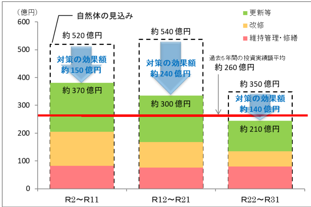
■図表 4-31 1年あたりのインフラ施設の平均必要額の経年推移（10年ごと）
