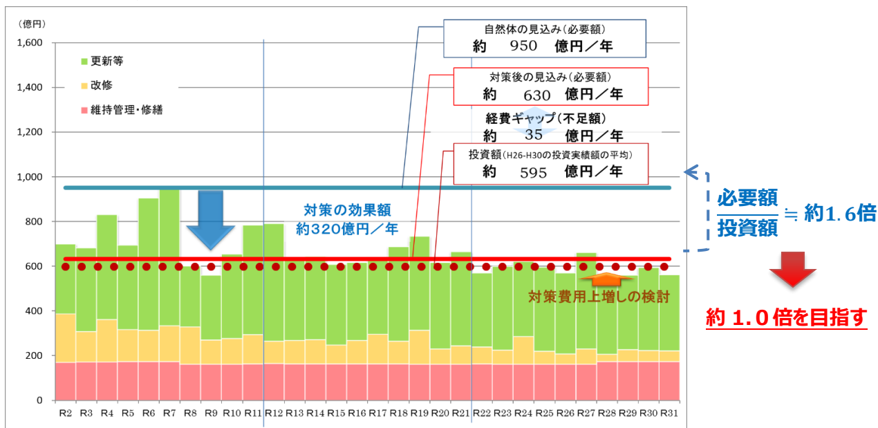
■図表 4-28 長寿命化等の対策を踏まえた（対策後の）見込み（30年間）
