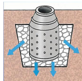
(浸透マンホールイメージ)
