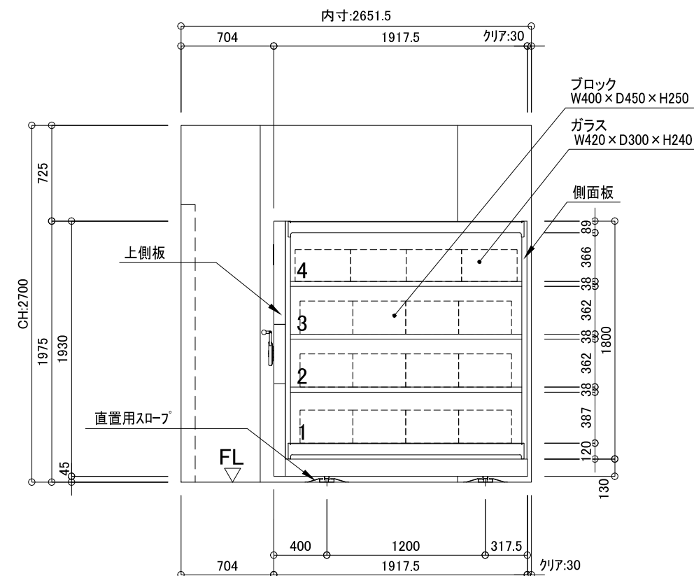
A側面図
