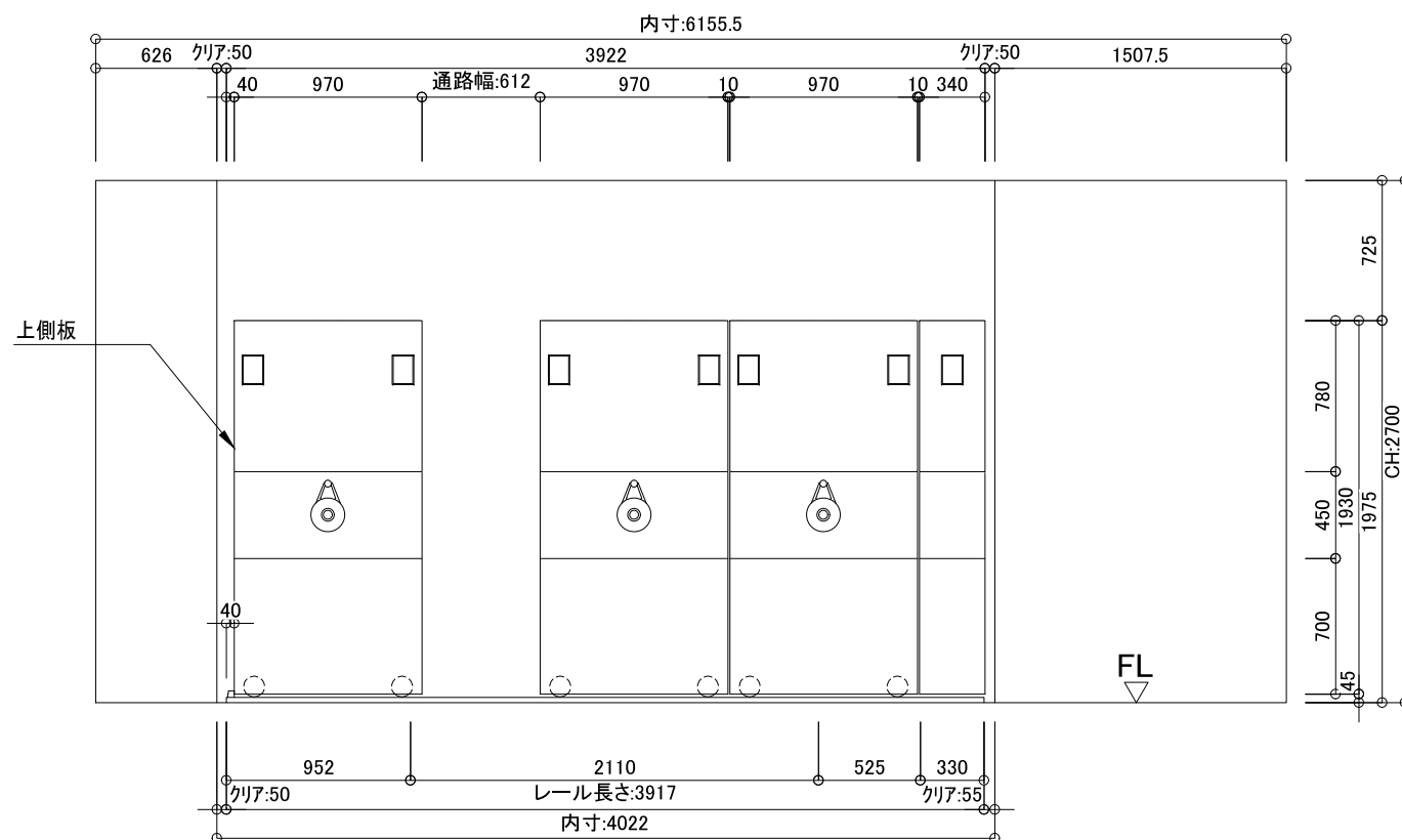
正面図
