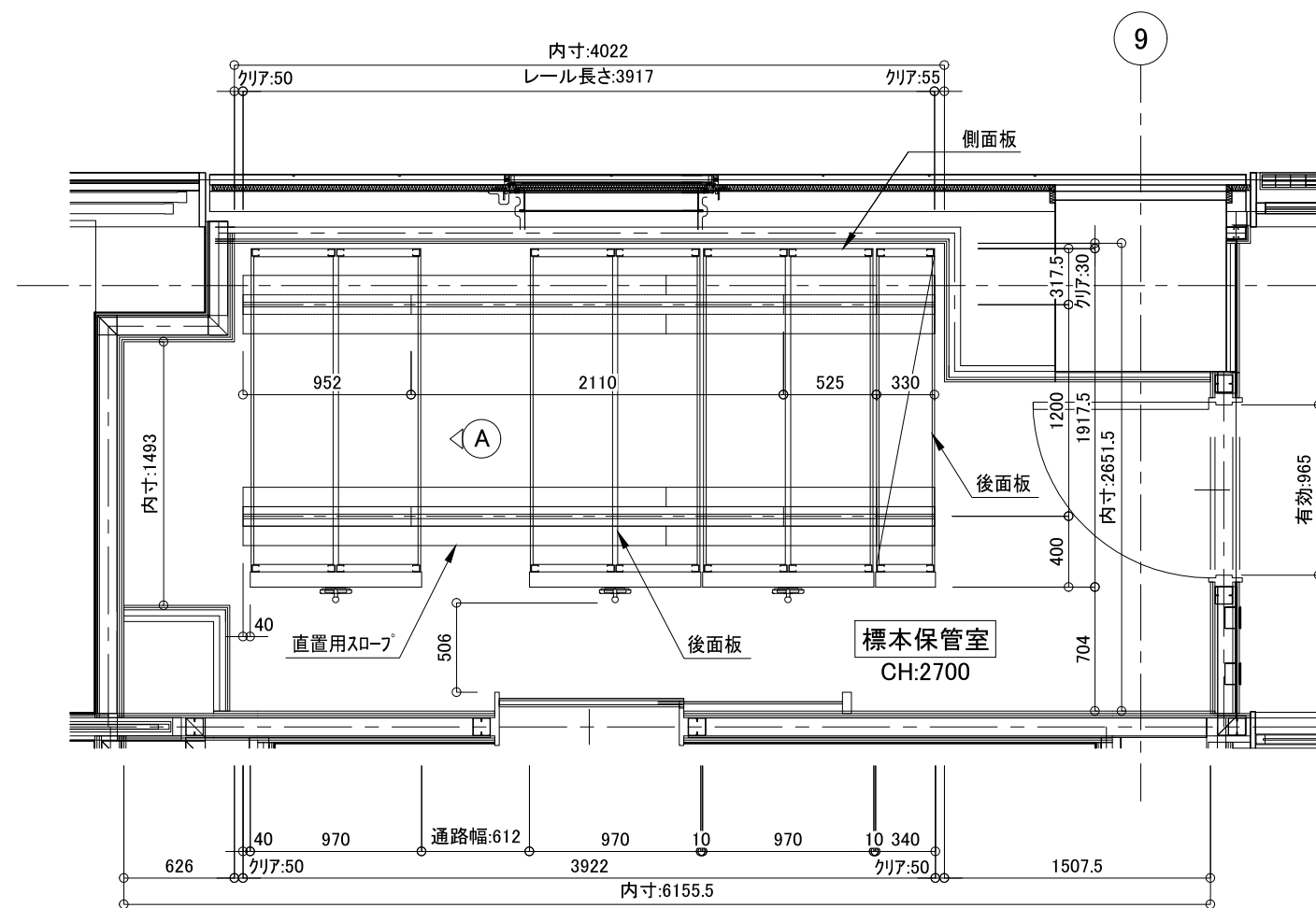
平面図
