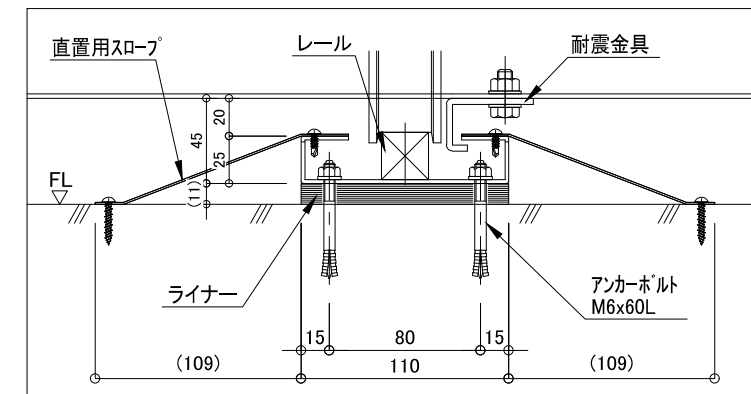
レール断面(直置き方式) S=1/20(A1) S=1/10(A3)
