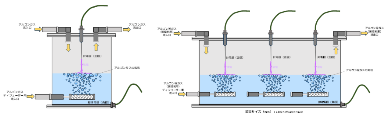
図 24 プラズマ処理で用いたリアクター（左：針電極 1 本リアクター、右：針電極 3 本リアクター）（No. W5）
