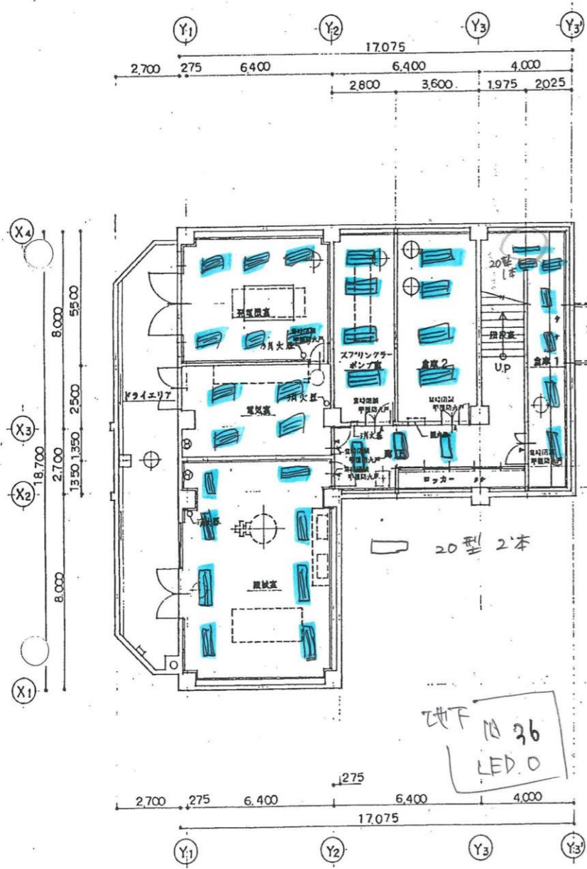
B1階平面図 Scale:1/100 凡例 240.73 m 2 ⊕: マンホールイモリ蓋600*を示す
