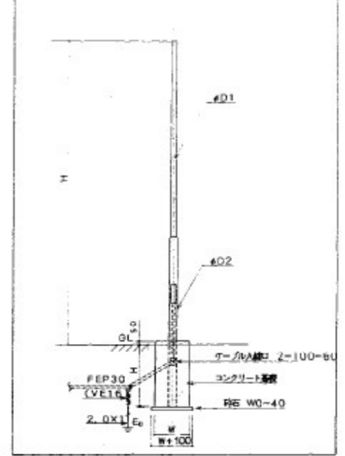
ポール詳細図
