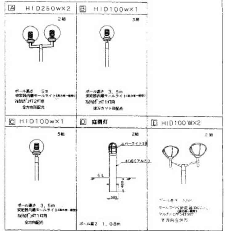
ポール詳細図
