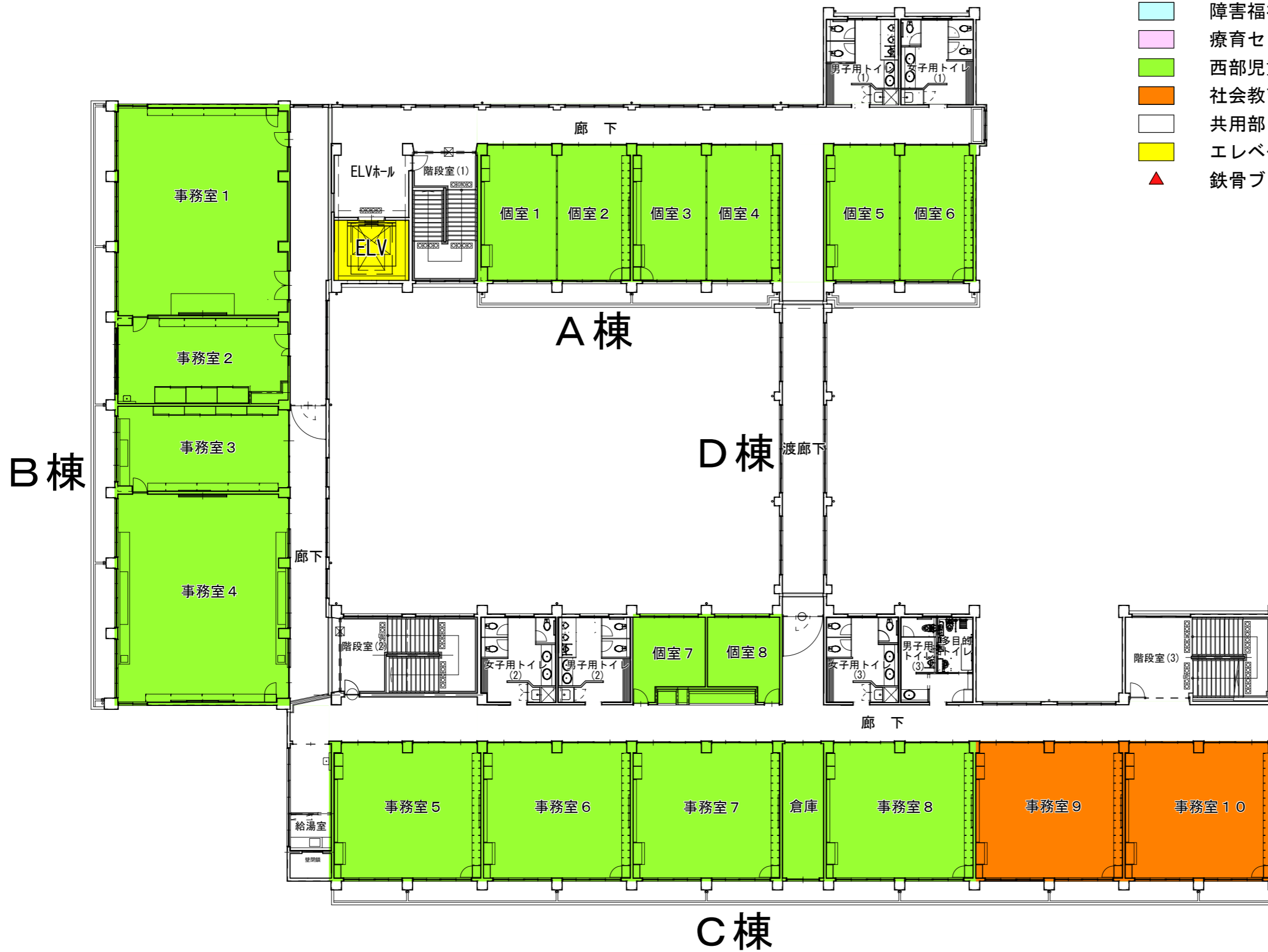
3階平面図
