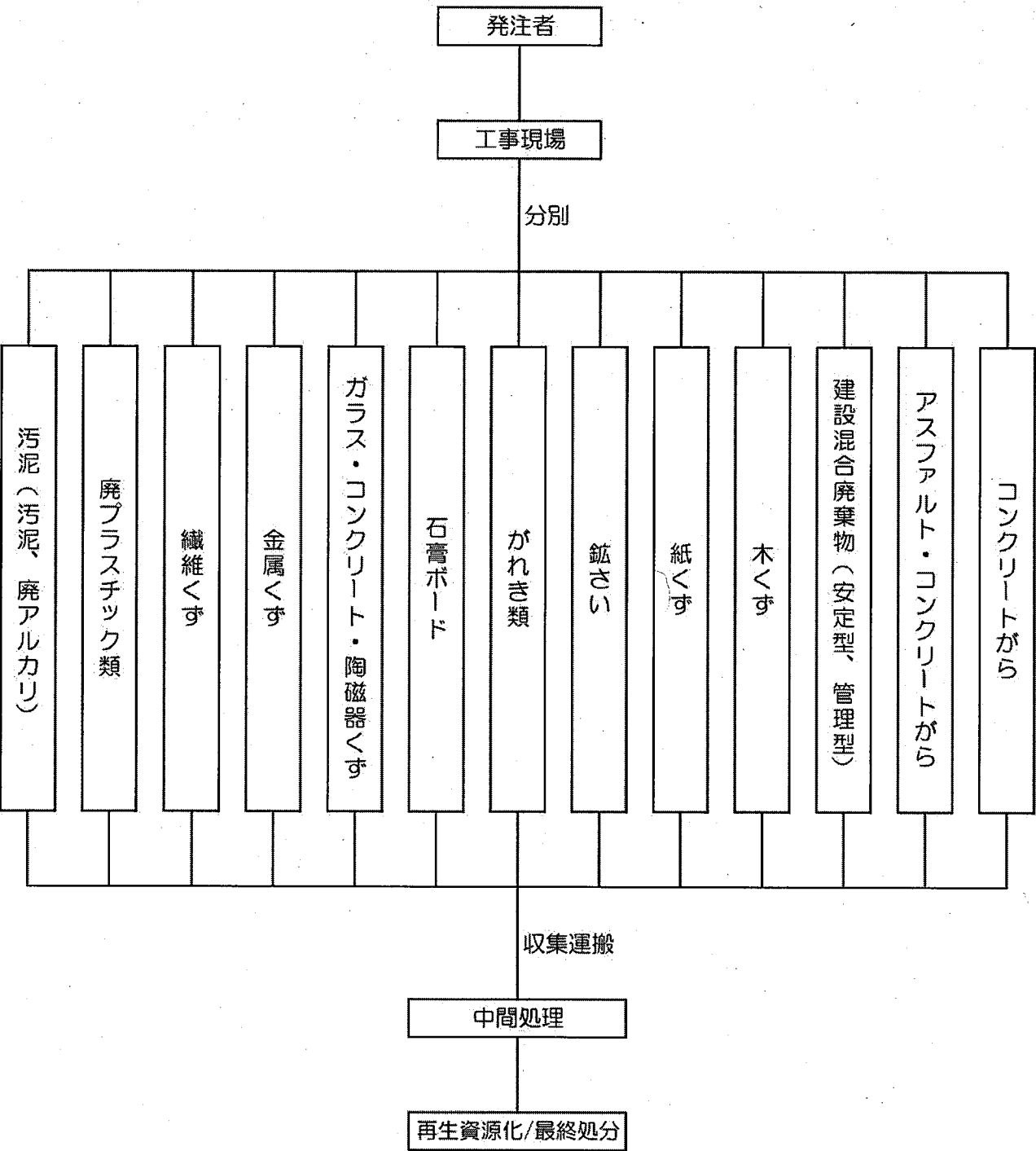
別紙1【処理工程図】
