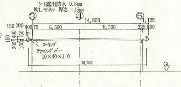
あ～あ 屋上断面図 S=1/200
