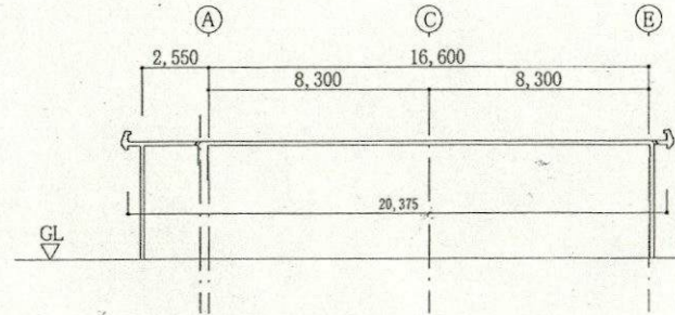
う～う 屋上断面図 S=1/200
