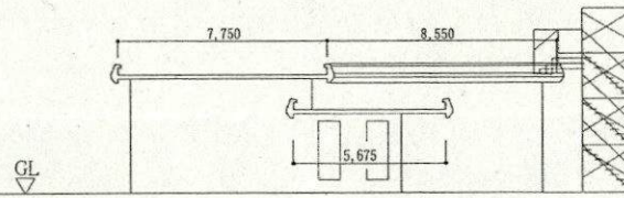
い～い 屋上断面図 S=1/200
