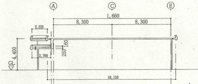
え～え 屋上断面図 S=1/200
