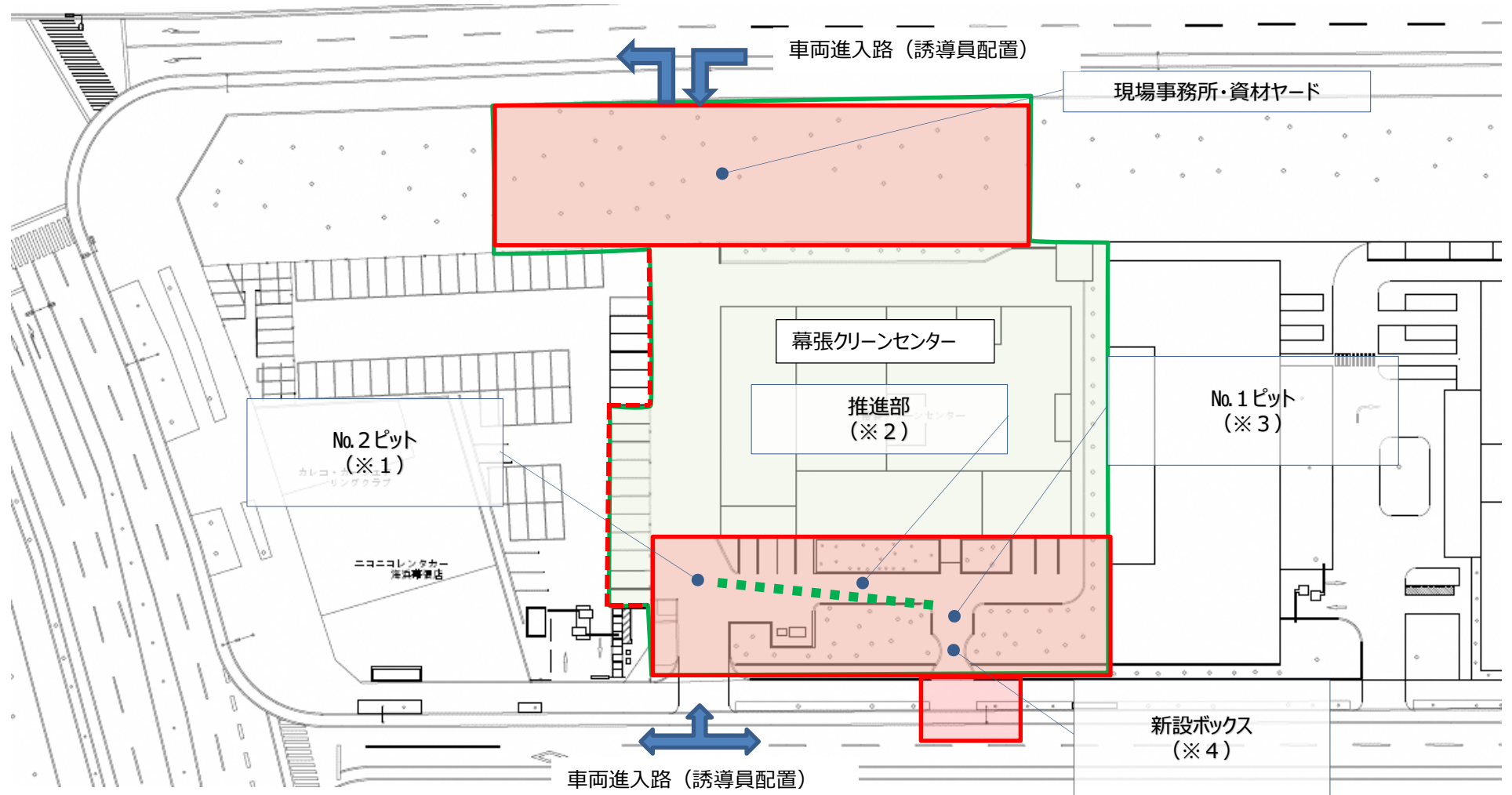
工 事 概 要 図
