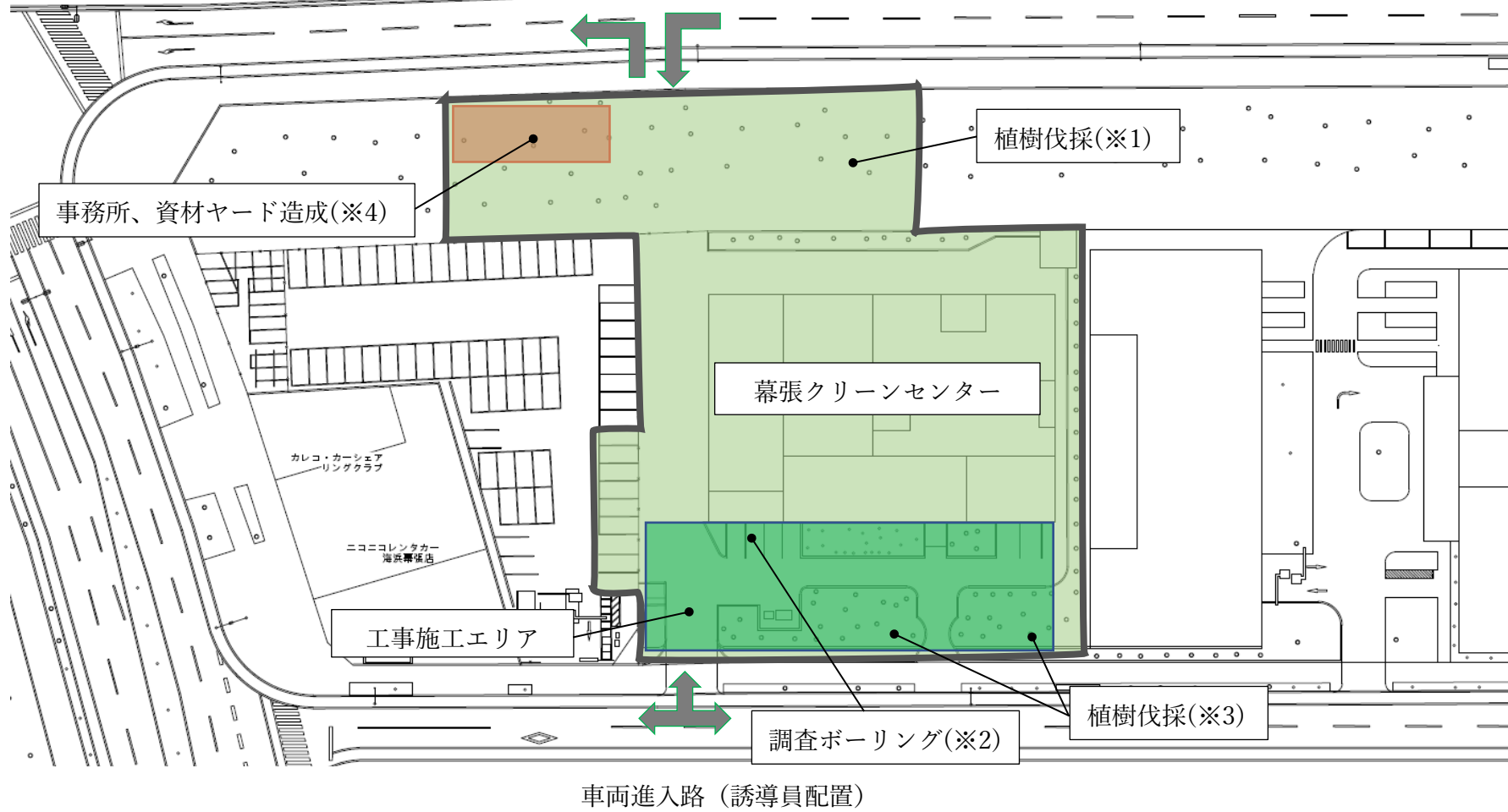
図1 工事概要図
