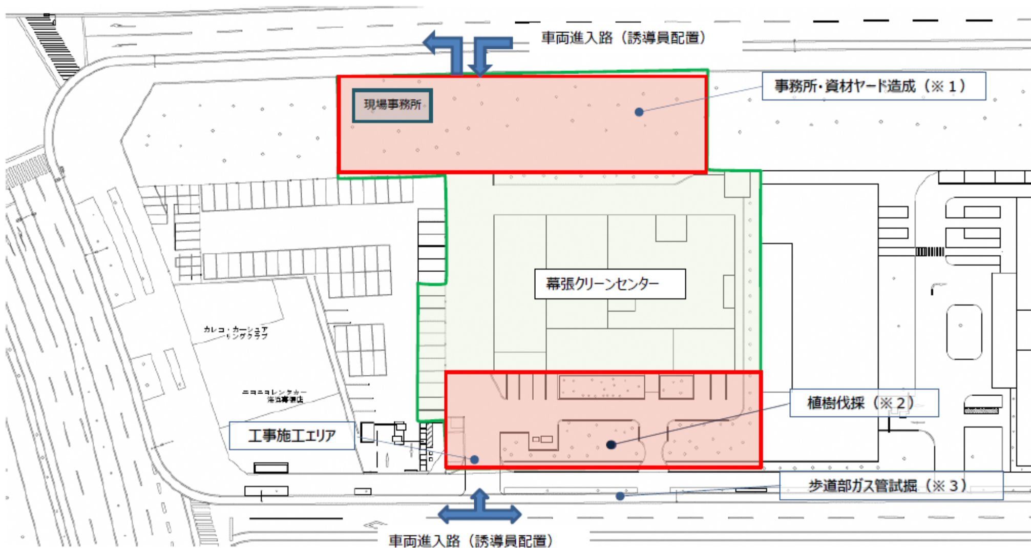
図 1 工 事 概 要 図
