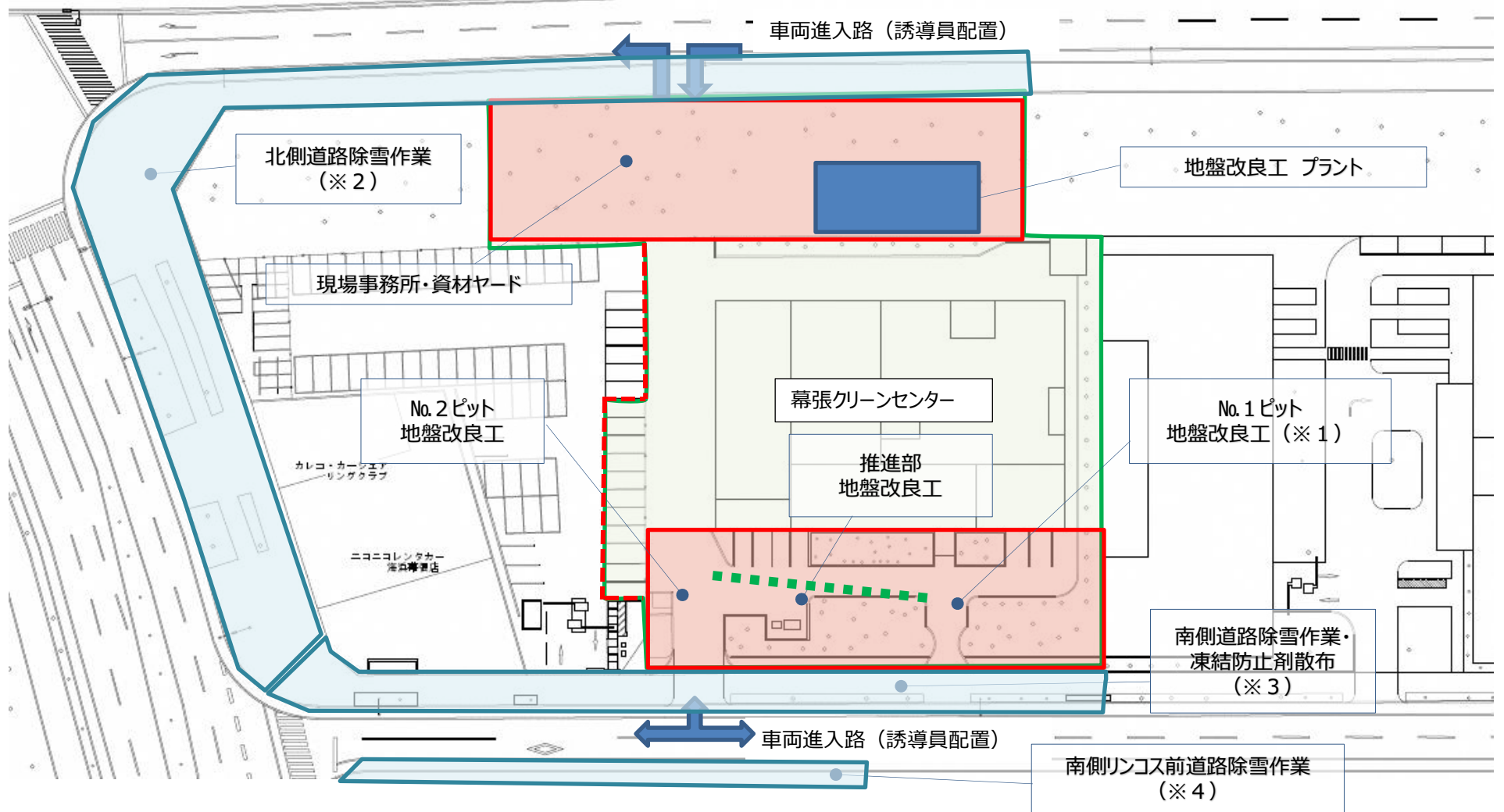
工 事 概 要 図
