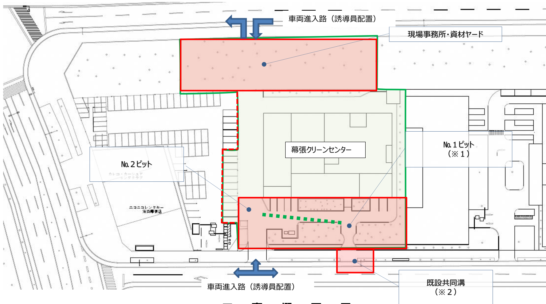
工事概要図
