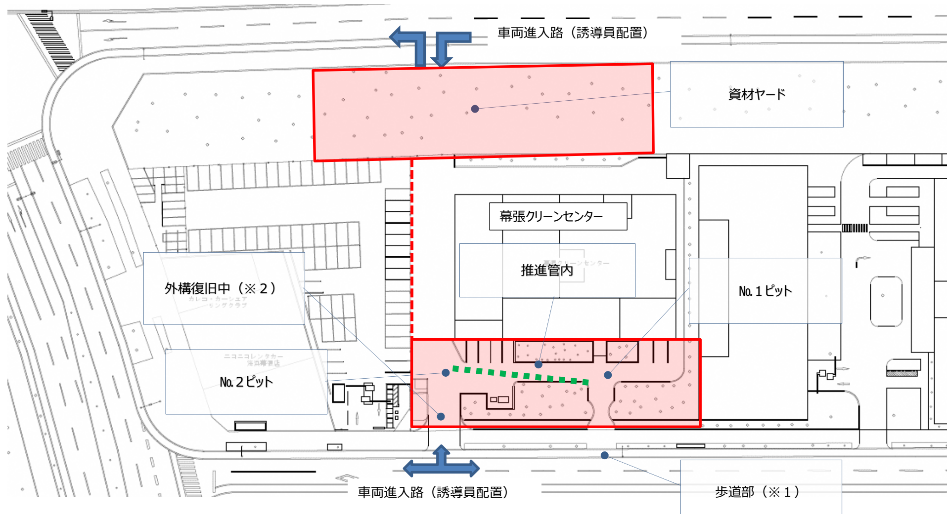
工 事 概 要 図
