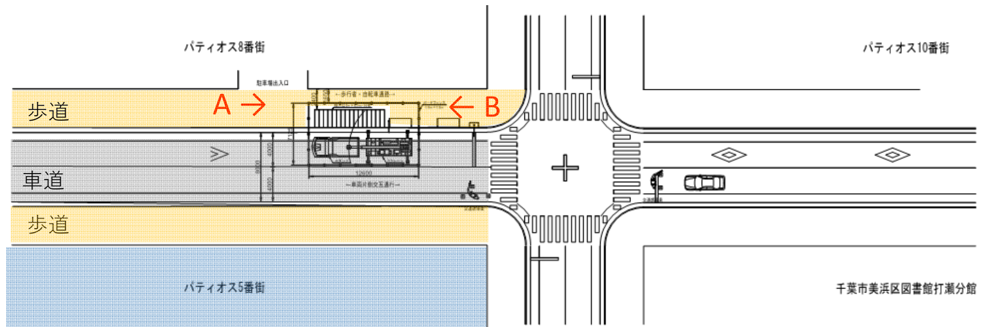
道路・歩道使用配置図
