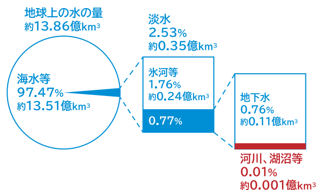
図 3-27 地球上の水の量
