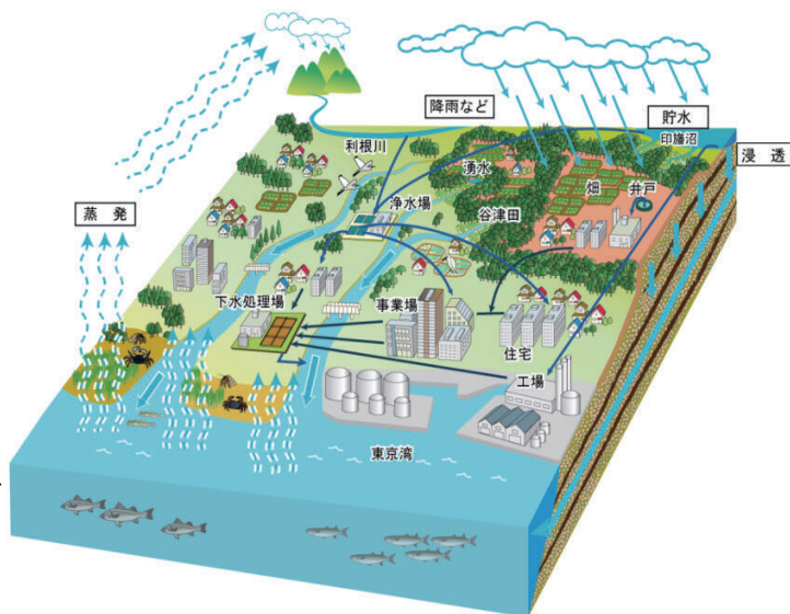
図 1-1 水循環の概念図
