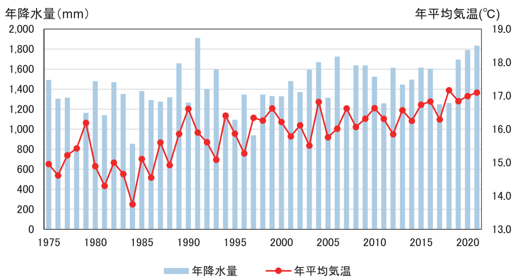
図 3-4 降水量・気温の変化
