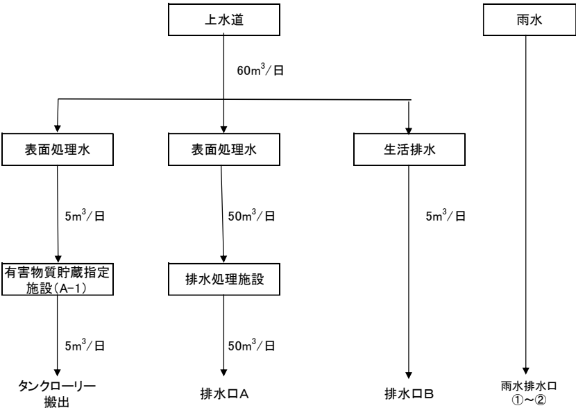
用水及び排水の系統図
