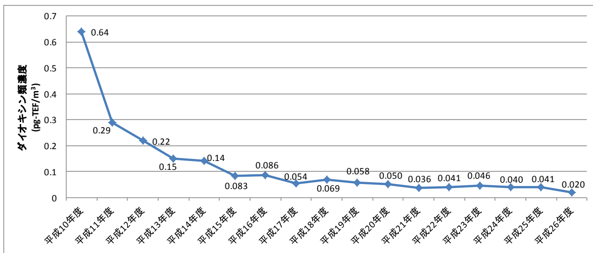
(参考) ダイオキシン類 全地点平均値の経年変化
