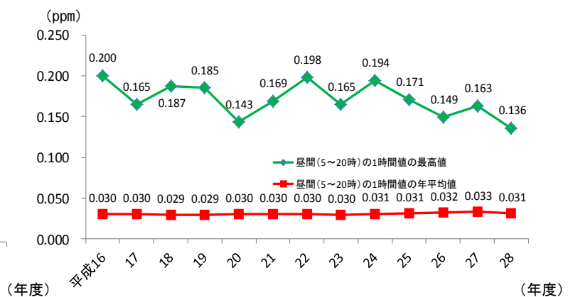
大気汚染測定局における昼間（5時～20時）の光化学オキシダント濃度
