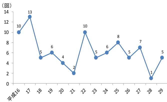
千葉地域における光化学スモッグ注意報発令回数
