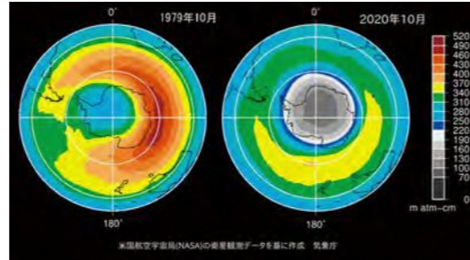
南極域のオゾンホールが現れる前の1979年(左)と2020年(右)それぞれの10月の平均オゾン全量の南半球分布。220m atm-cm(白色)以下の領域がオゾンホール。米国航空宇宙局(NASA)提供の衛星データをもとに気象庁が作成。
