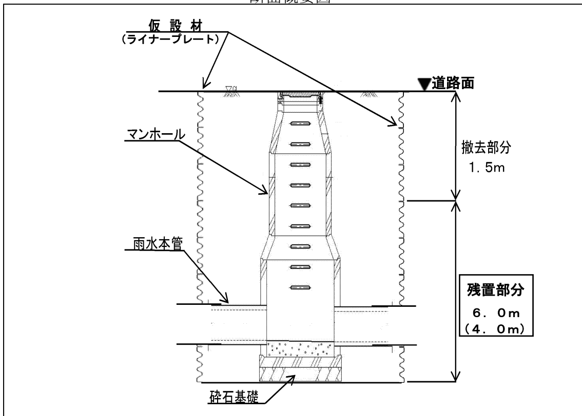
断面概要図
