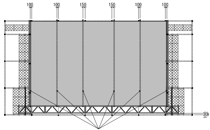
単管 L6000 平面図 (シート取付図)
