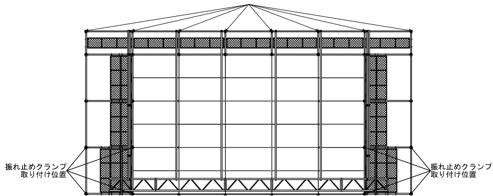
振れ止めクランプ取り付け位置
