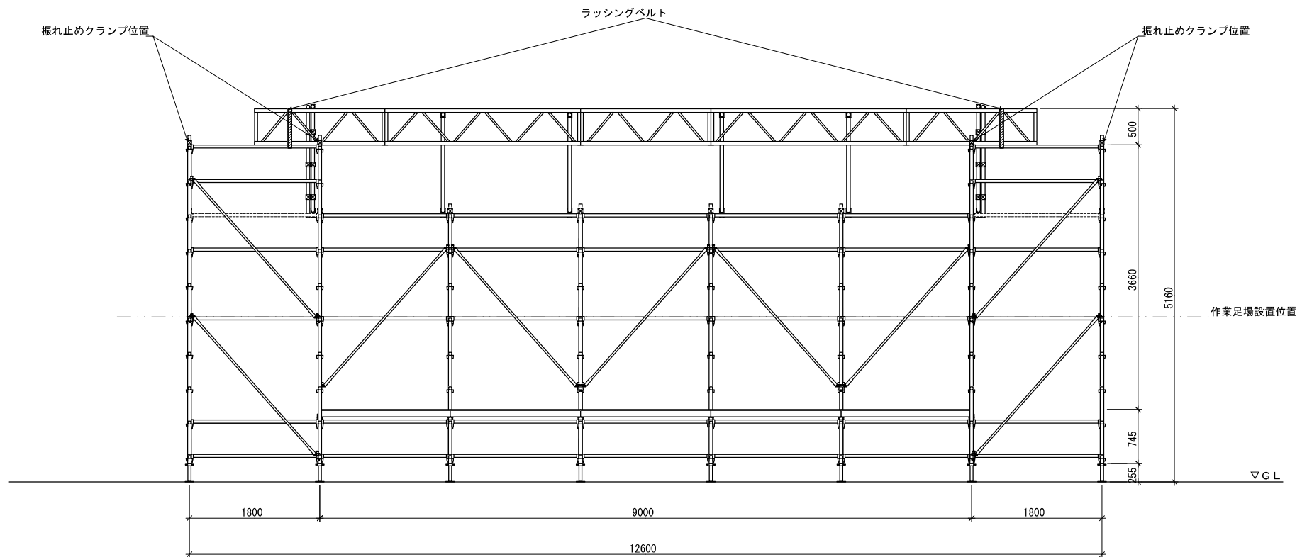
立面図
