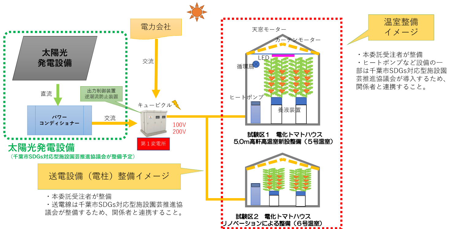
(図2)再生可能エネルギーを活用したトマト施設栽培実証イメージ
