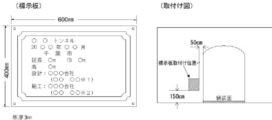
図 6-2 標示板の設置イメージ図
