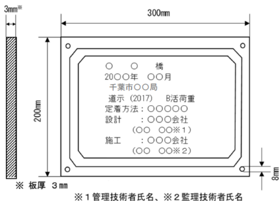
図2-2 銘板の寸法及び記載事項
