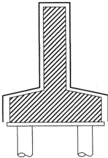
図-1 擁壁
