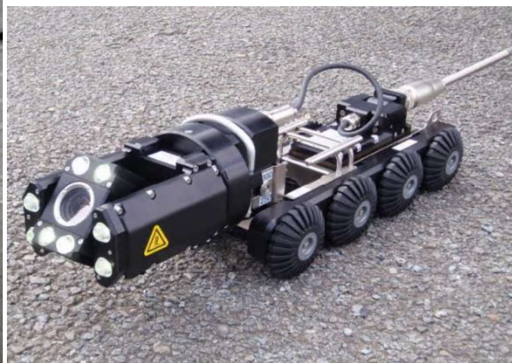
【TVカメラ】
