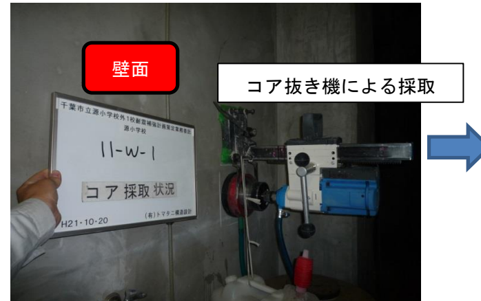
コンクリート壁のコア採取
