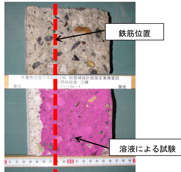
中性化試験
