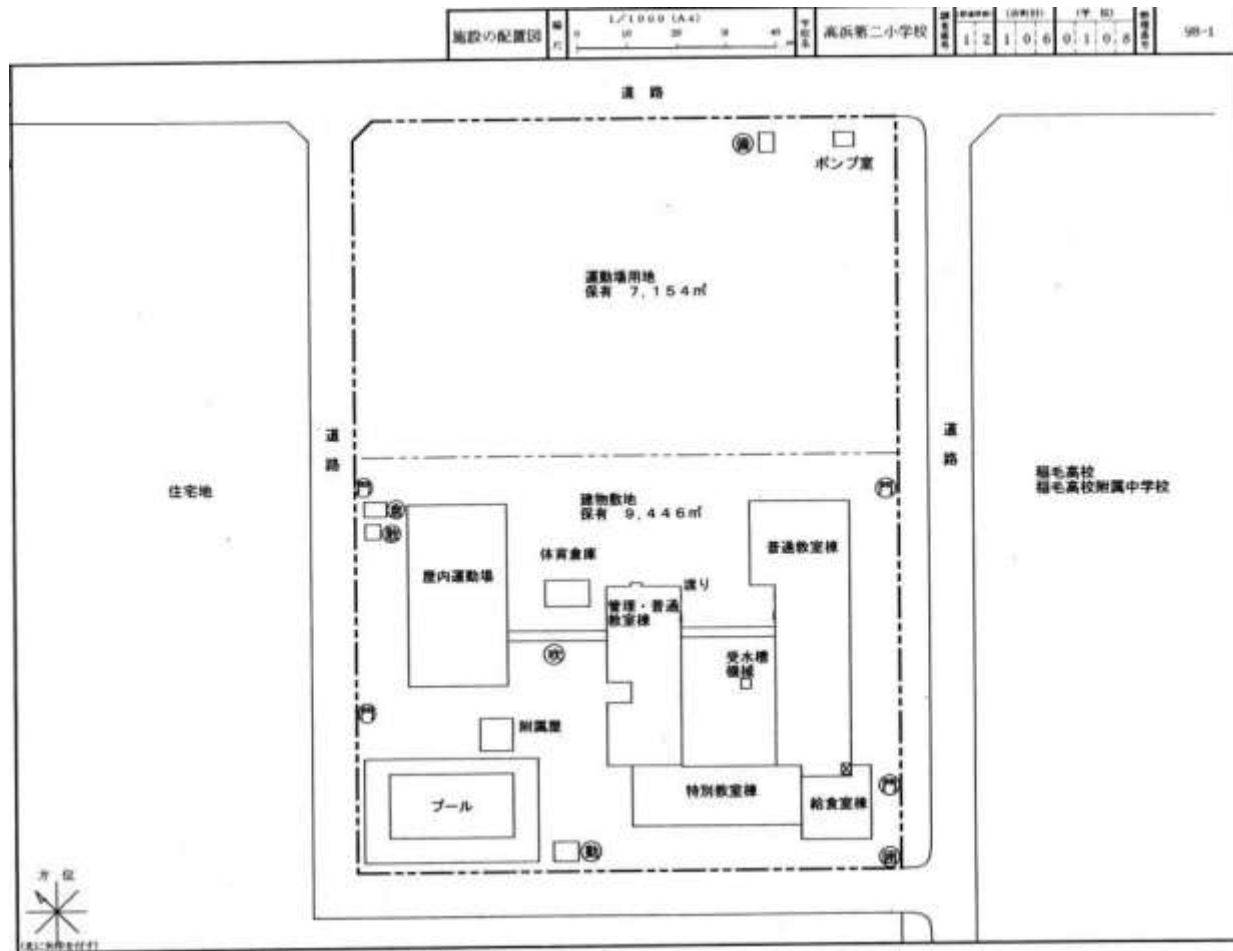
3 高浜第二小学校校舎配置図
