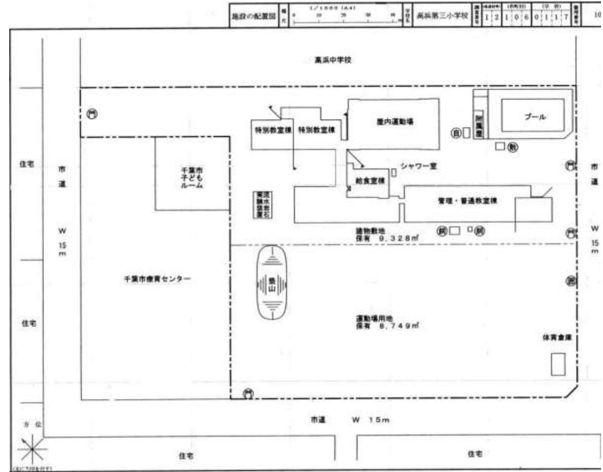
4 高浜第三小学校校舎配置図
