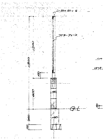
A-A' 断面図 1/20
