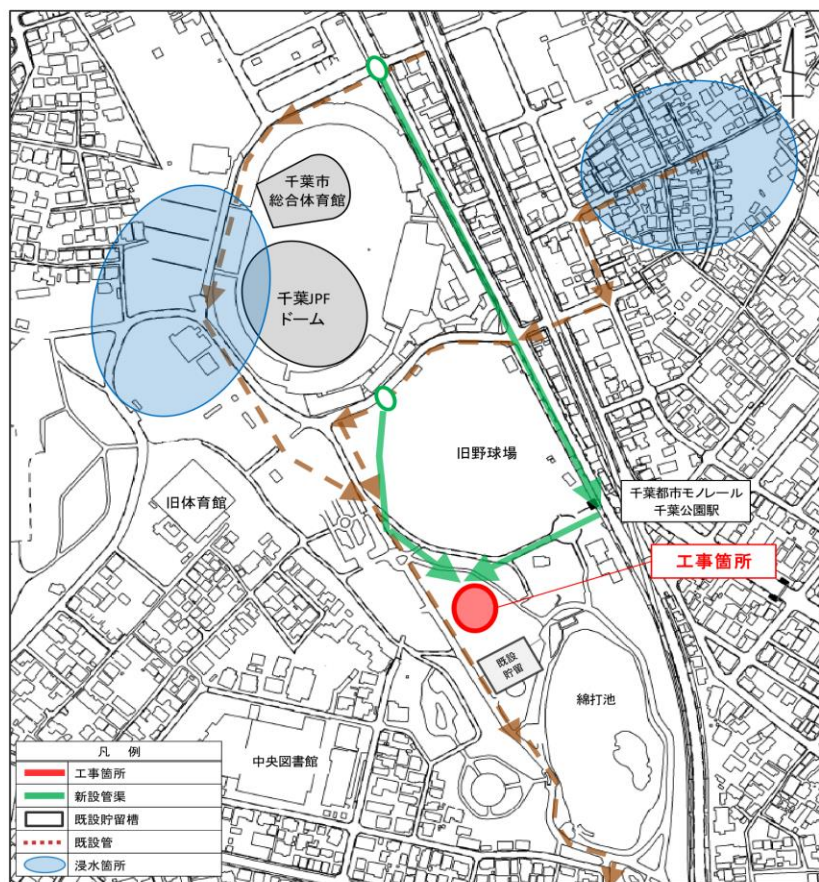
雨水貯留槽位置図（参考）
