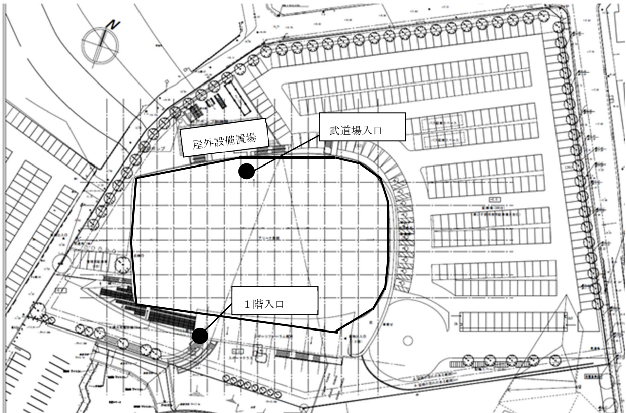
【案内図】
