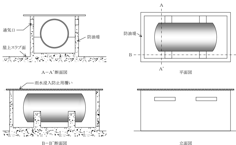
例図3 中継タンクの防油堤概略図
