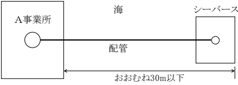
第3-11-2図 移送取扱所に該当しない例（その2）
