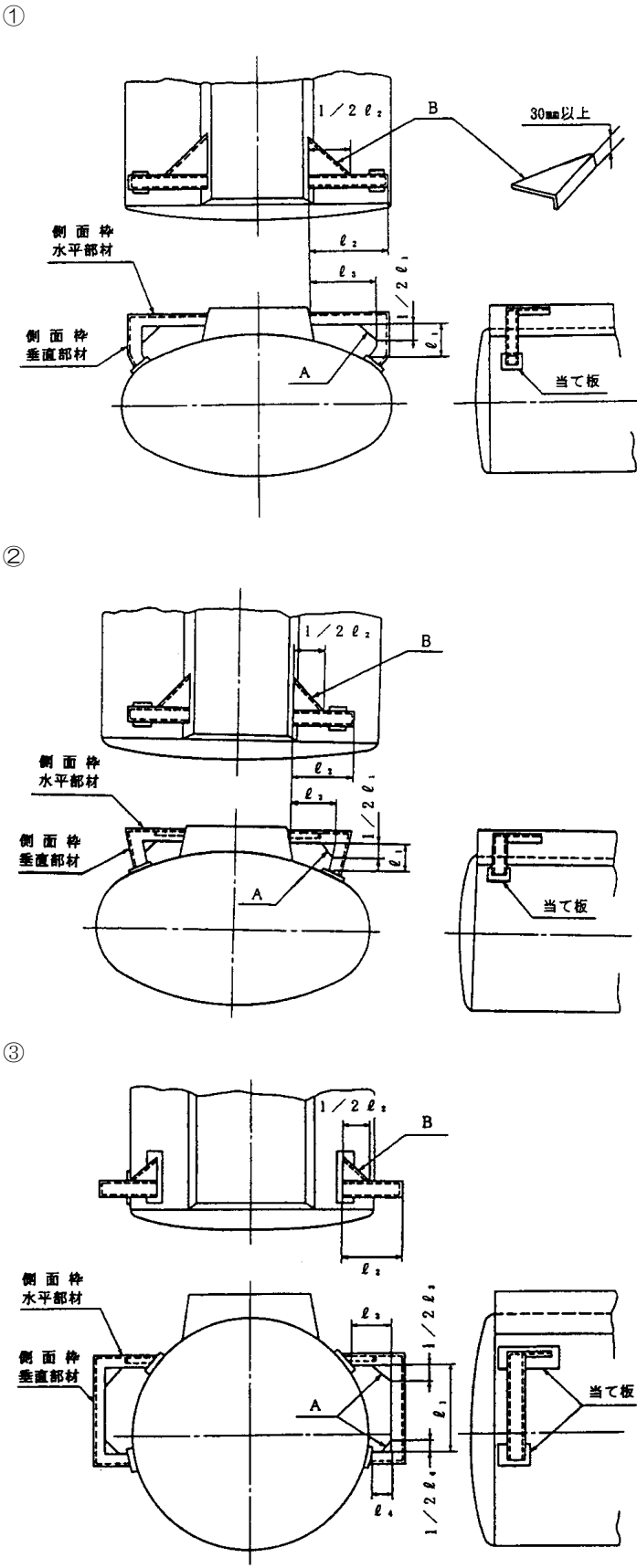
第3-7-10図 枠形の側面枠の構造
