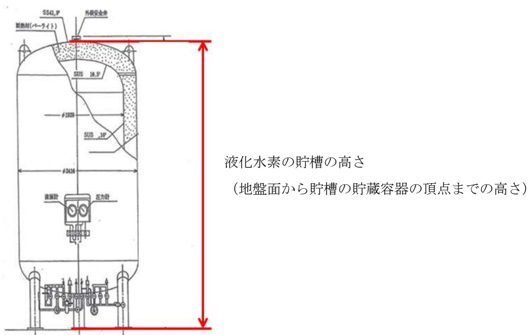
第3-9-49図 液化水素の貯槽の高さ
