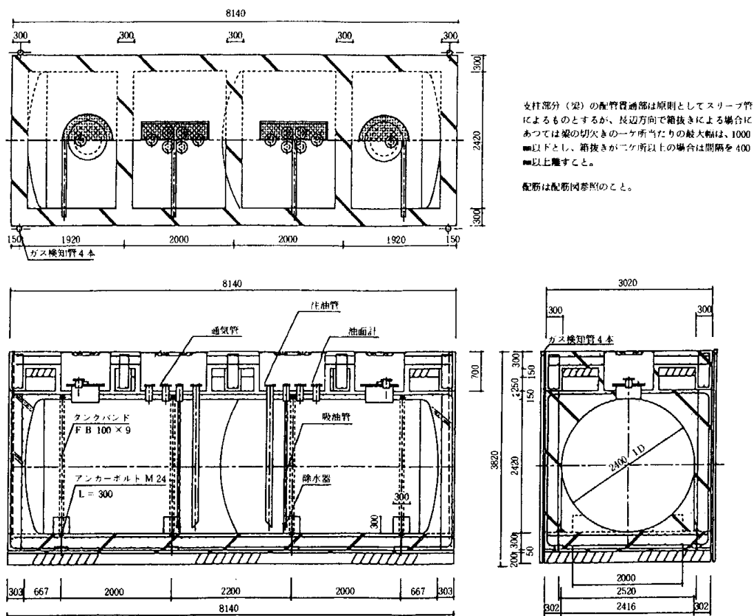
コンクリート被覆タンク配筋図
