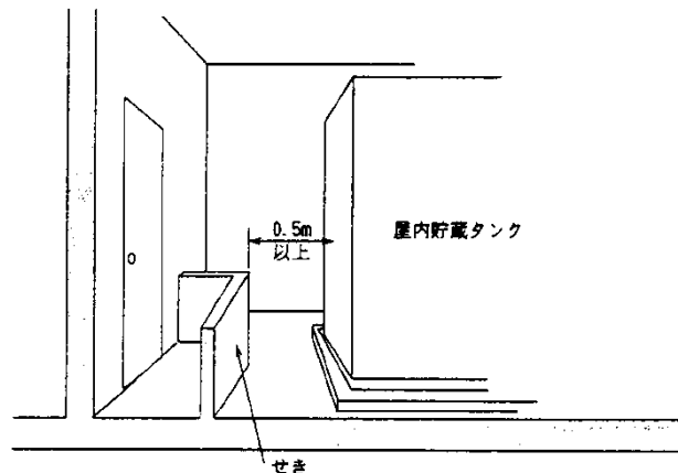
第3-4-1図 セきを設ける例
