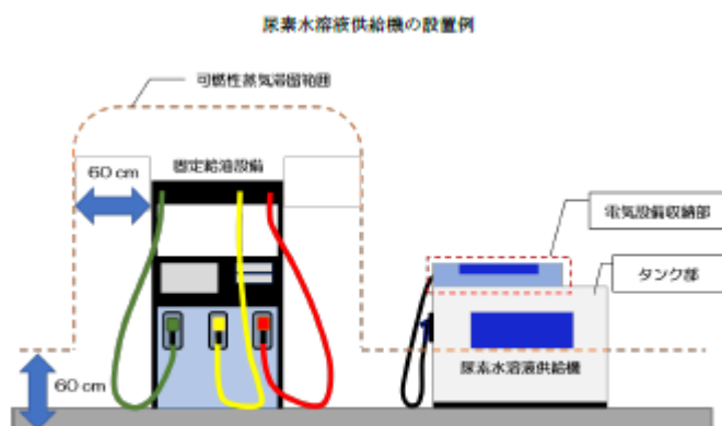
図1 尿素水溶液供給機（電動ポンプにより払い出すタイプ）
