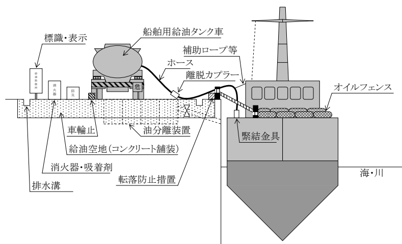
(立面図)
