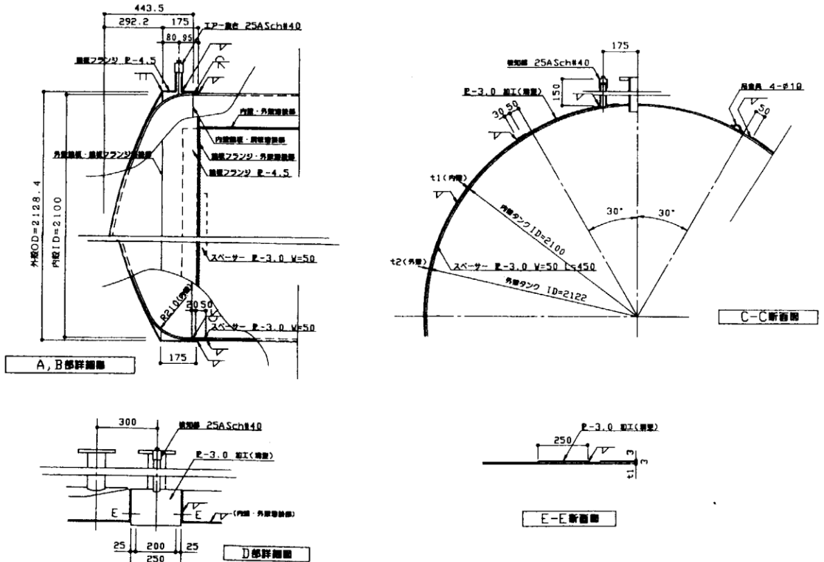
第3-5-13図（その4の2） 鋼製二重殻タンク各部の例（25kL 内径：2100）
