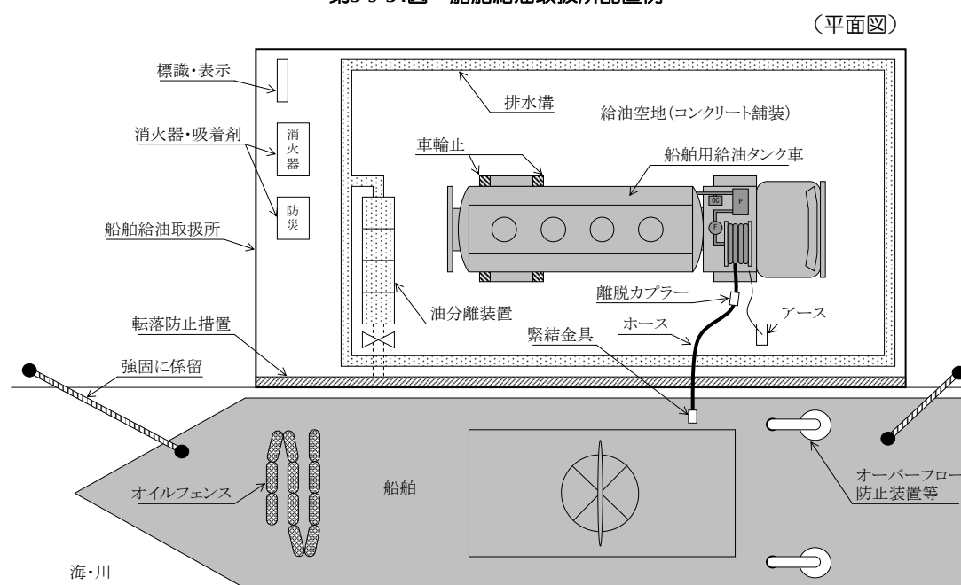
第3-9-34図 船舶給油取扱所配置例
