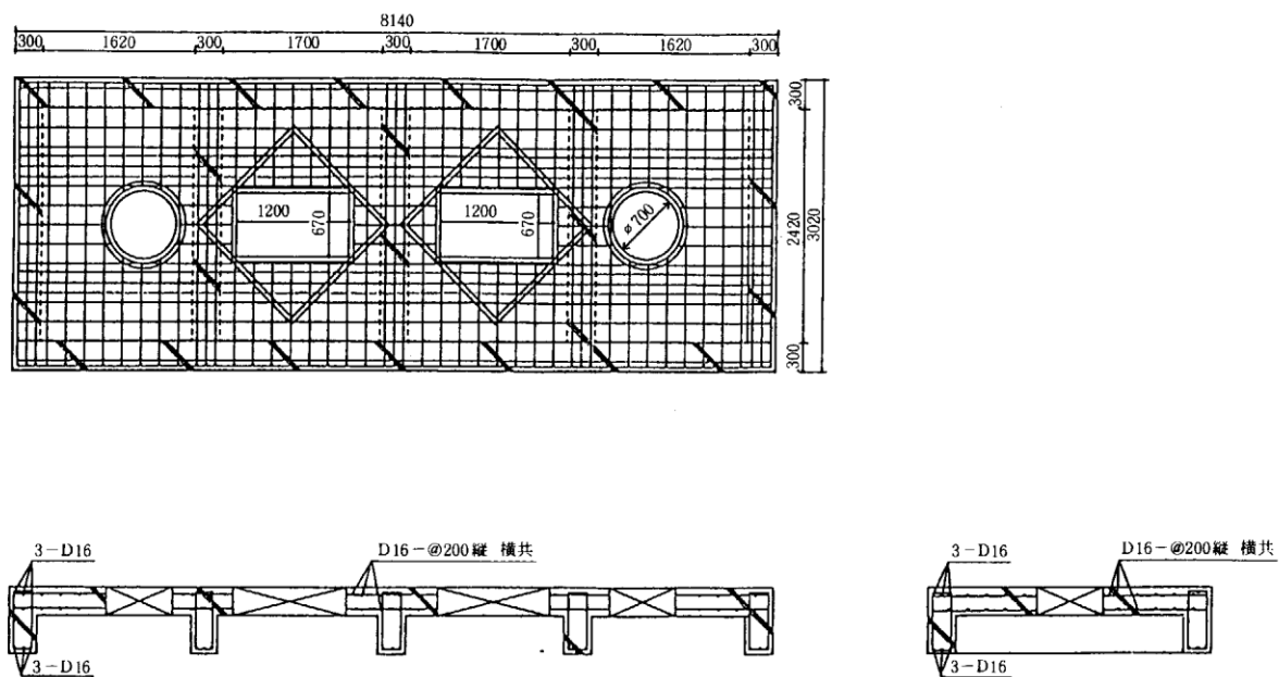
コンクリート被覆タンク配筋図
