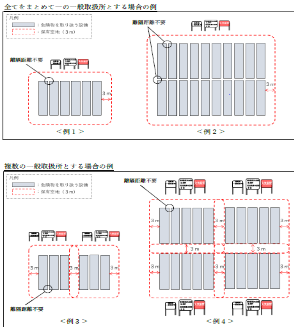
第 3-12-8 図 屋外コンテナ等蓄電池設備の設置例
