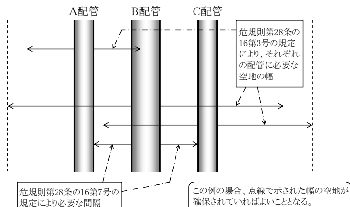
第3-11-7図 配管の両側に保有すべき空地
