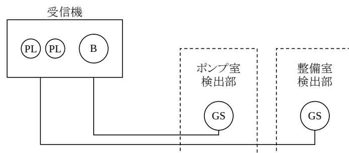
第3-9-28図 可燃性蒸気検知警報設備の系統例
