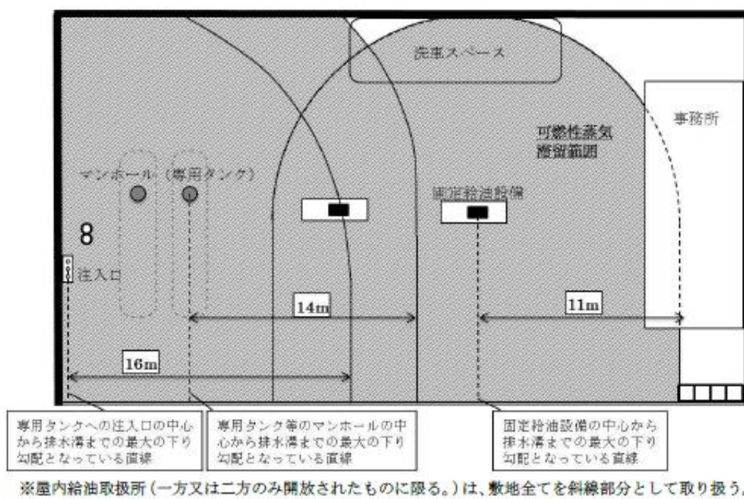
図4 給油取扱所（平面図）
