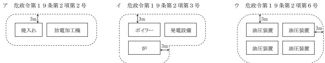
第3-12-3図 複数の設備を一の一般取扱所として規制する例
