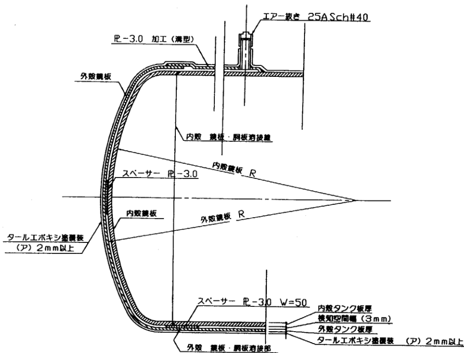
第3-5-12図（その5） 鋼製二重殻タンクの鏡板部断面詳細
