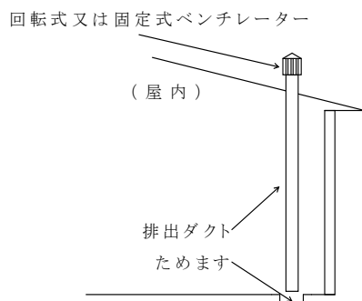
第3-1-11図 自動強制排出設備の例
