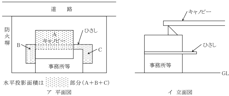
第3-9-2図 水平投影面積の算定例
