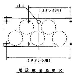
第3-5-14図（その3） 漏れ検知装置の例（5タンクの場合）
