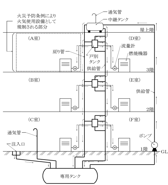
例図 2-2 中継タンクを有する方式の燃料系統図（系統例2）
