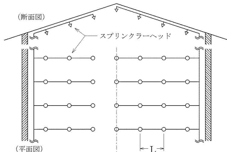
第3－7図 正方形又は矩形配置の場合
