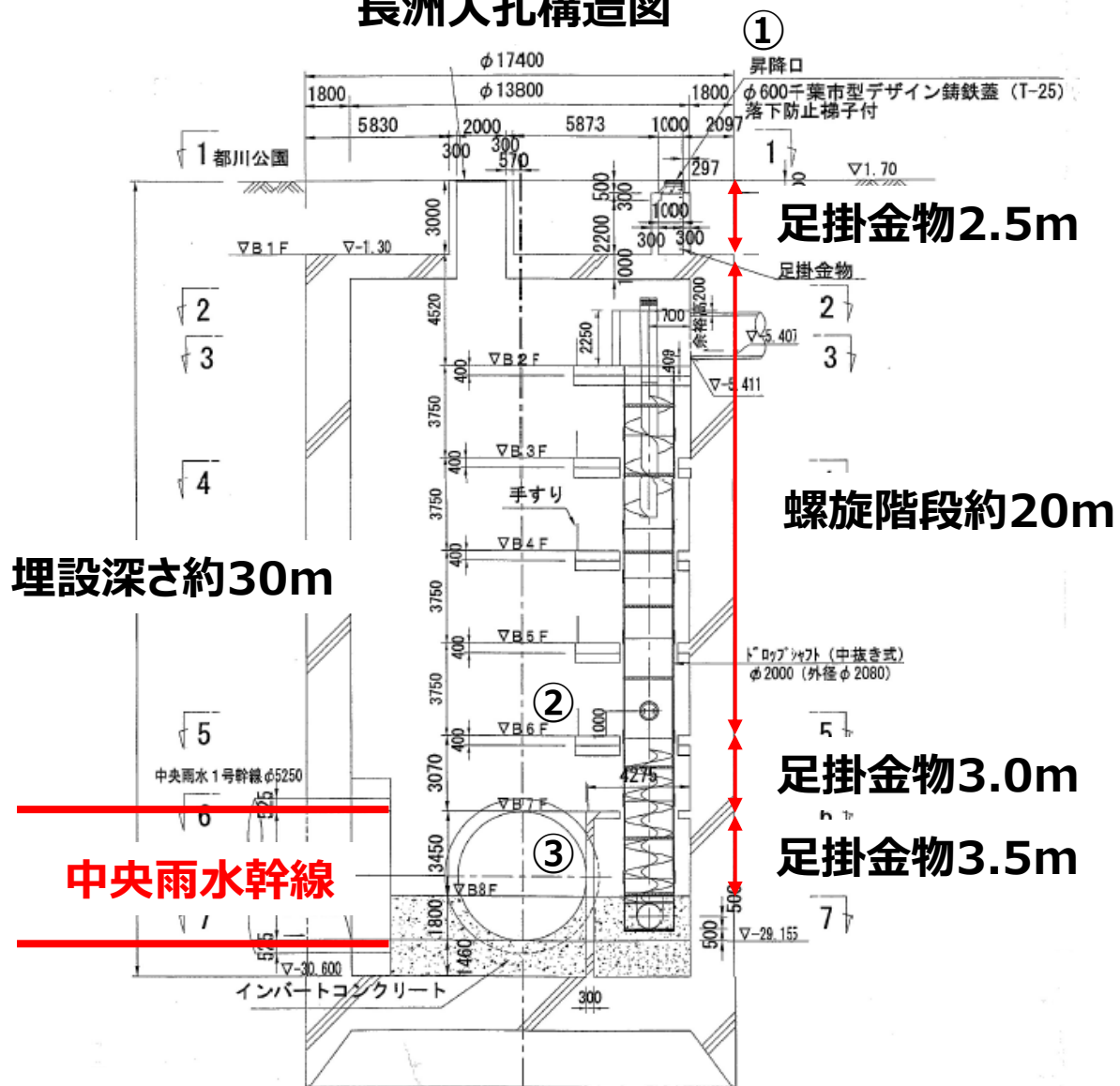
長洲人孔構造図
