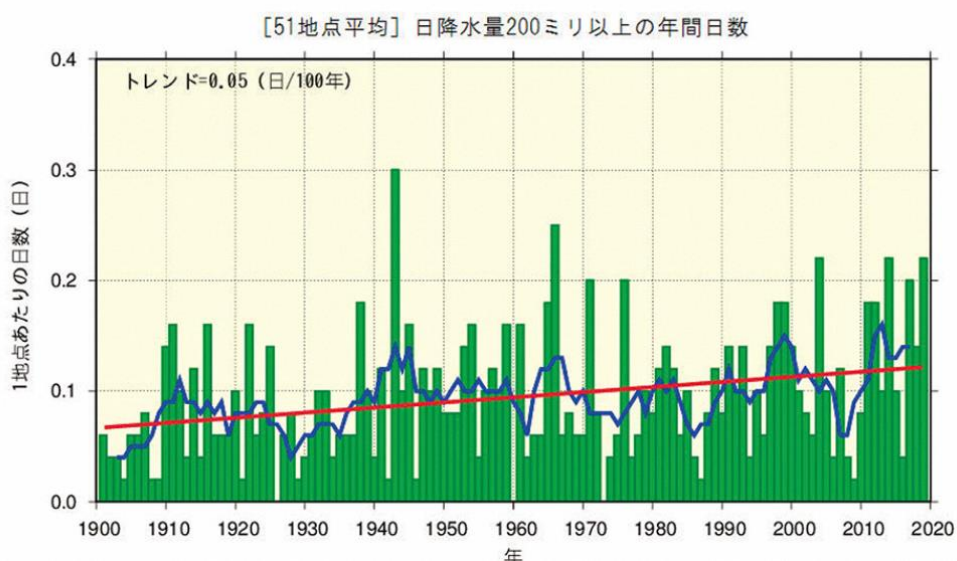
図 2-26 日降水量 200 ミリ以上の年間日数の推移 出典：気象庁
