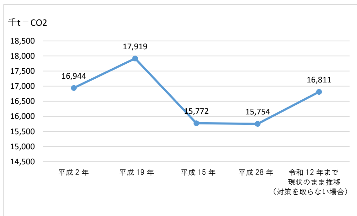
図 2-25 千葉市の温室効果ガス排出量
