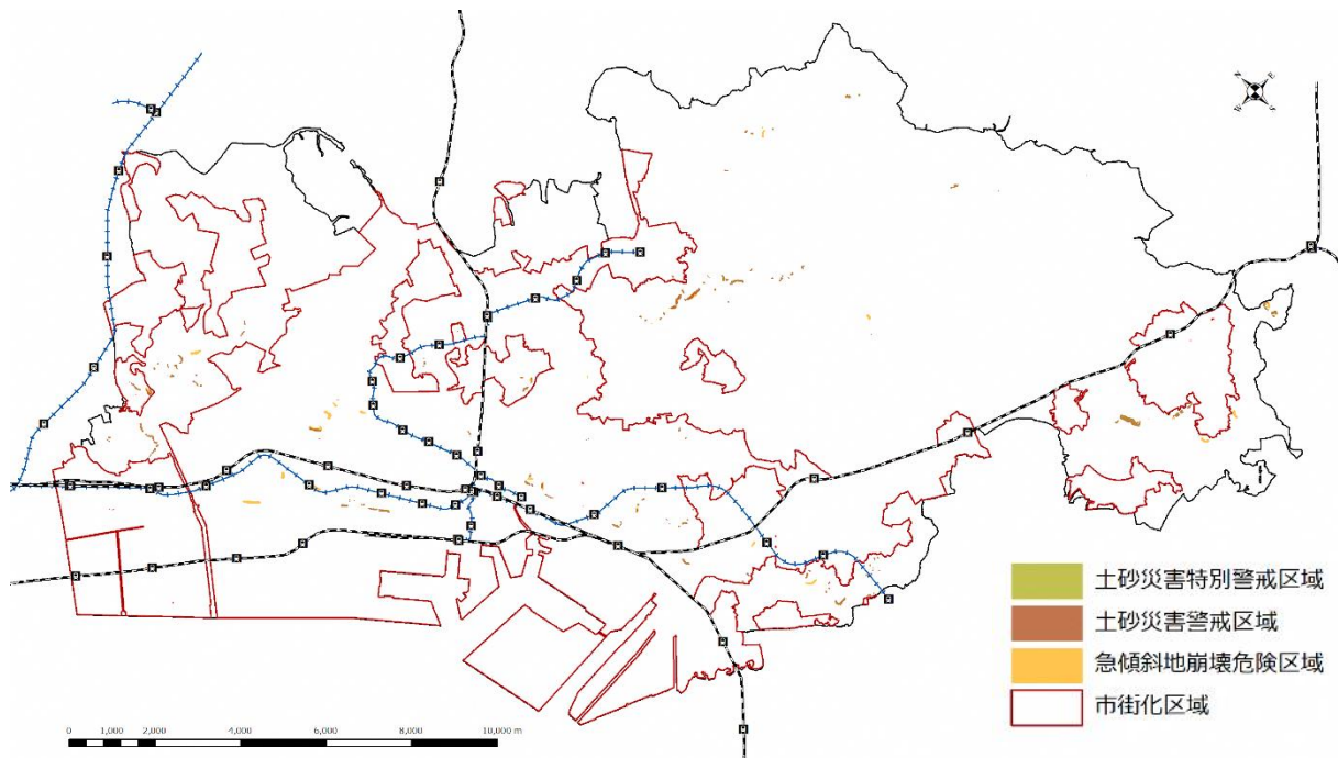
図 2-69 土砂災害特別警戒区域
