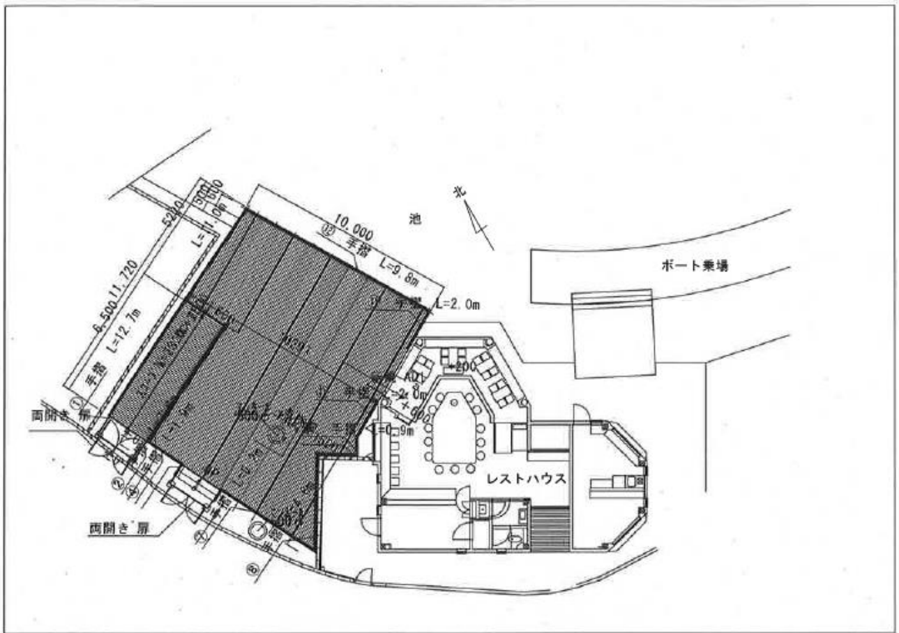
平面配置図
