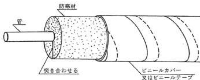
図 3.7-2 防寒材
