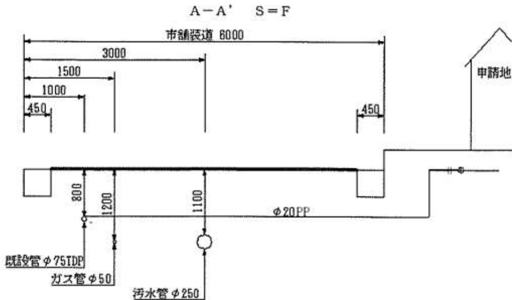
道路埋設断面図
