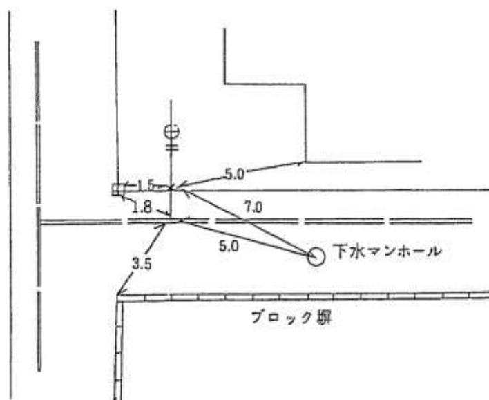
図 6.3-1 分岐位置、第 1 止水栓及び標示杭等のオフセット標準図
