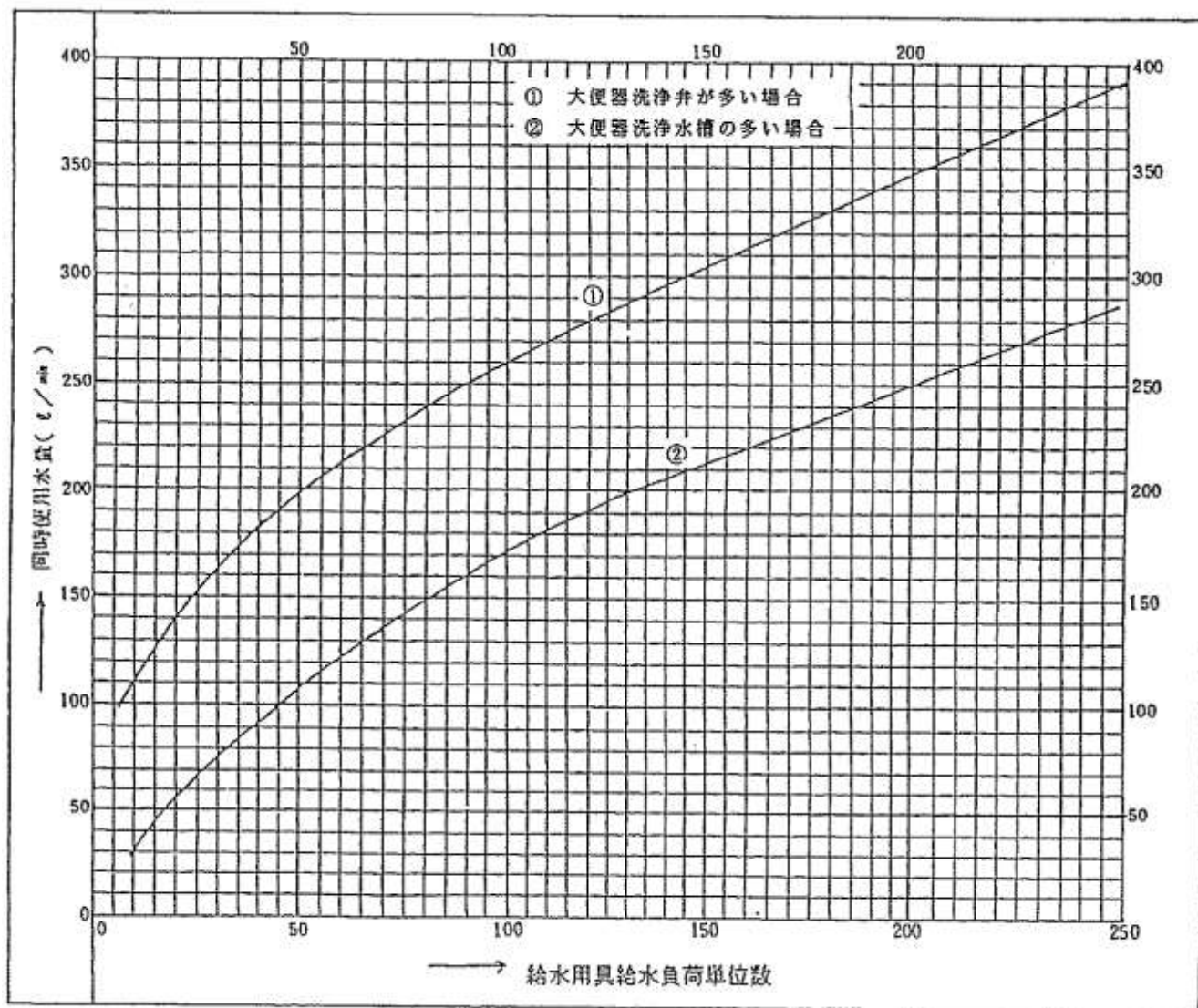
図 2.4-1 給水用具給水負荷単位による同時使用水量図 (給水用具給水負荷単位数 0~250)
