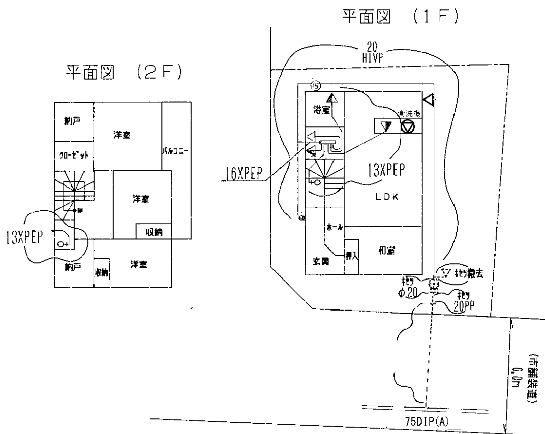
図 6.1-1 平面図標準図
