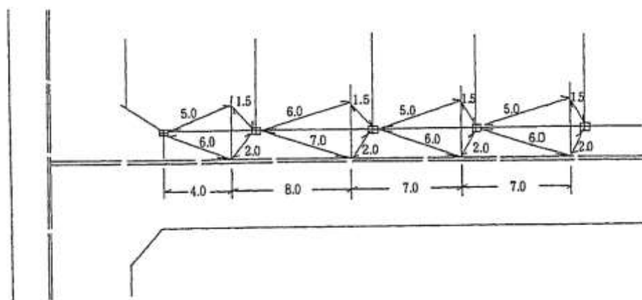
図 6.1-4 一部先行工事のオフセット標準図
