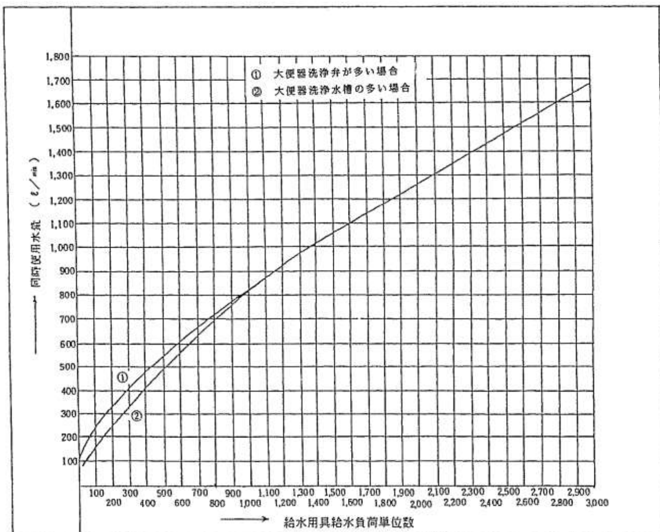
図 2.4-2 給水用具給水負荷単位による同時使用水量図（給水用具給水負荷単位数 0～3000）
