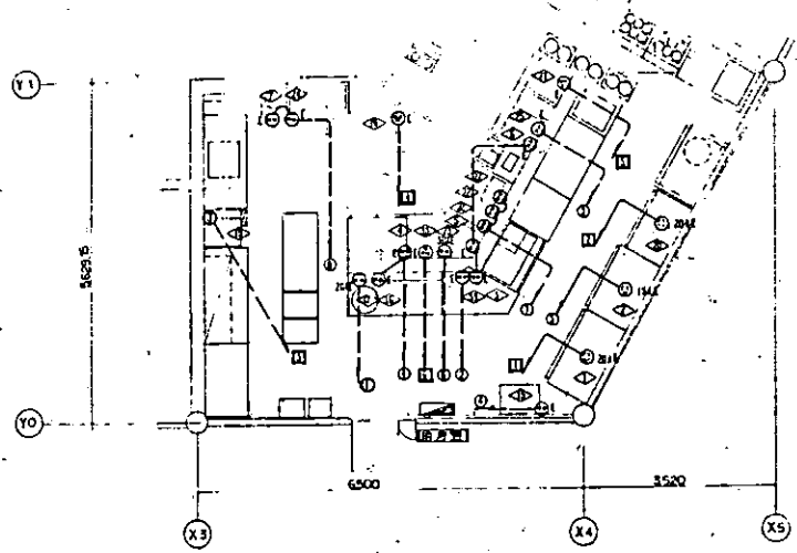
厨房コンセント図 S-1/50
