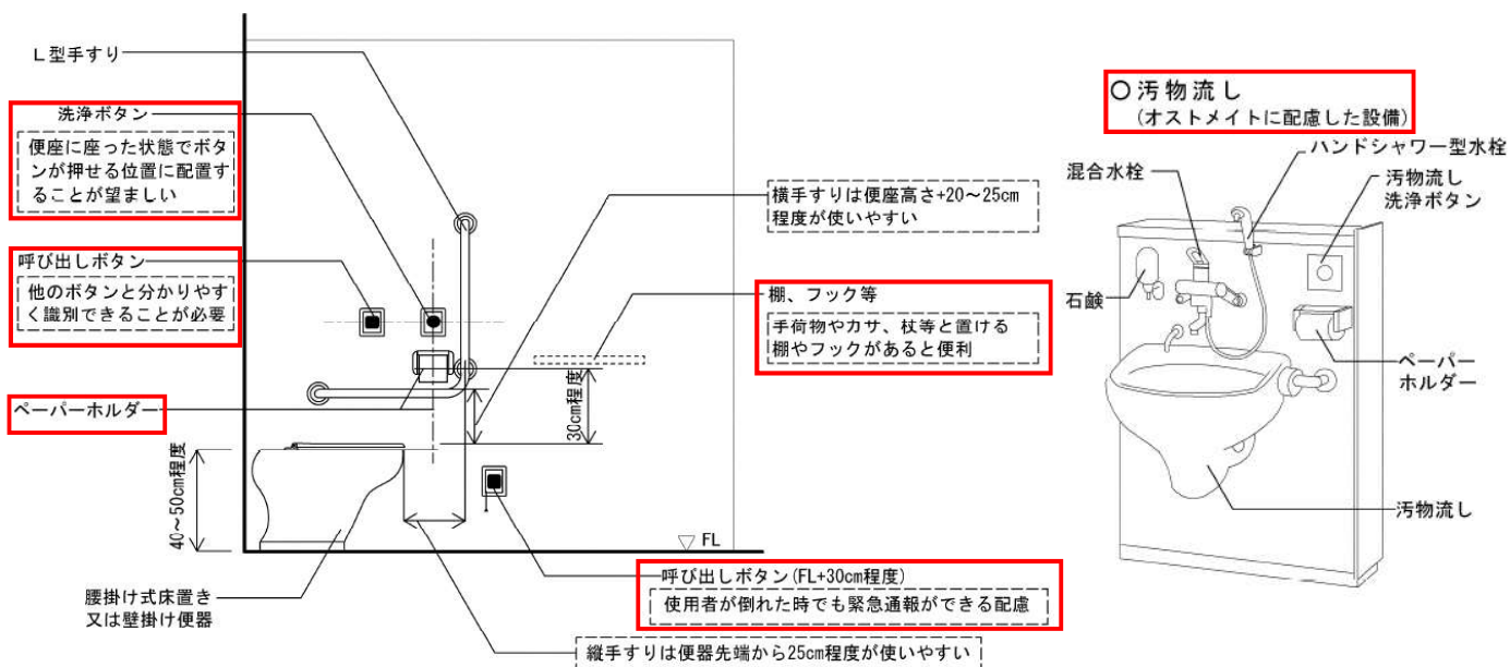
図 43 トイレのバリアフリー化（車椅子対応・機能分散）
