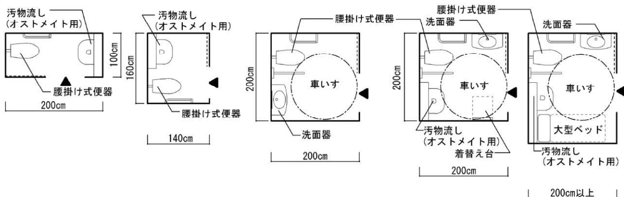
図 44 トイレのバリアフリー化（ボタン等の配置）
