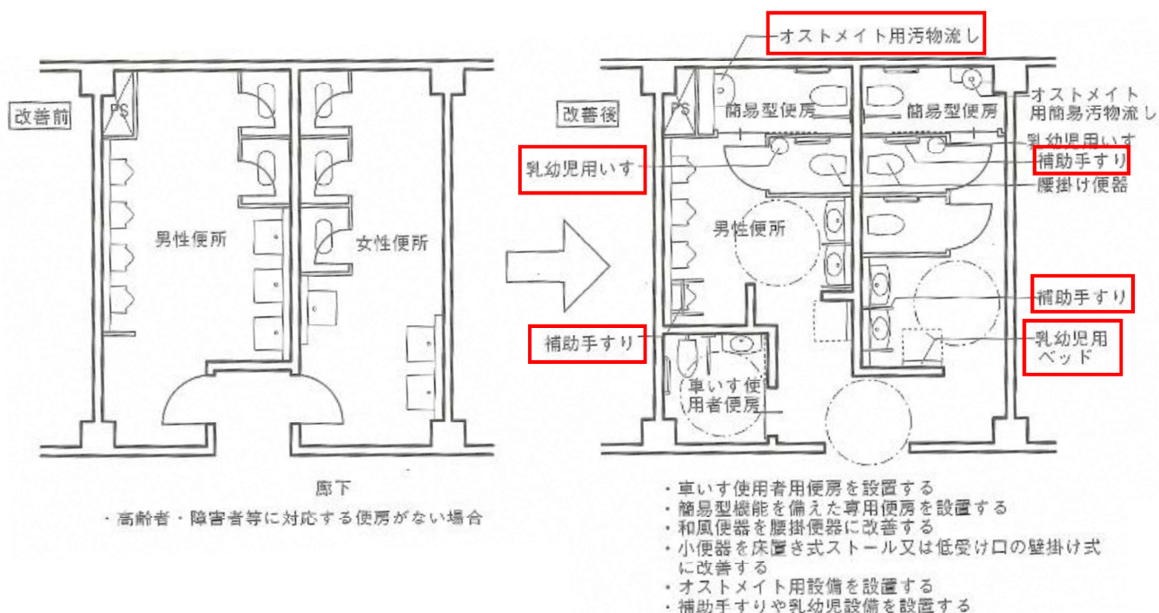
図 43 トイレのバリアフリー化（車椅子対応・機能分散）
