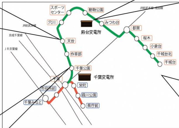
軌道桁を自営線として活用
