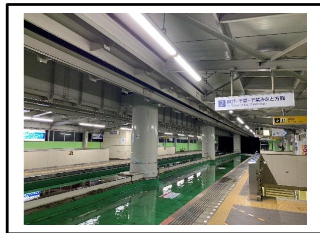
小倉台駅(2021(R3)年度施工)
