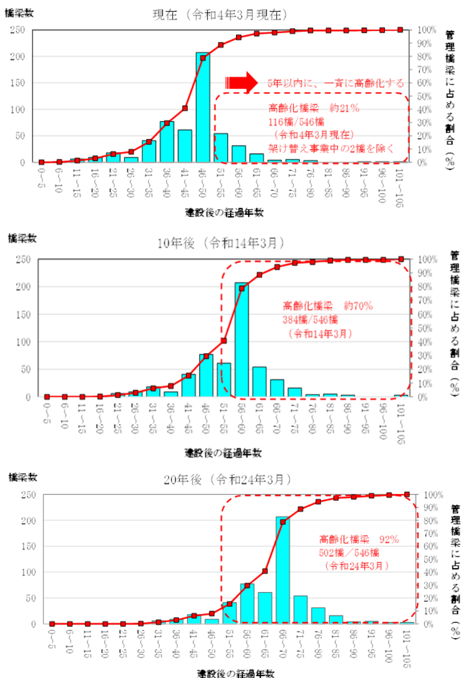
■図表 2-18 橋梁の例 架設後経過年数別の橋梁数の分布
