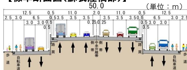
【標準断面図(蘇我陸橋部)】
